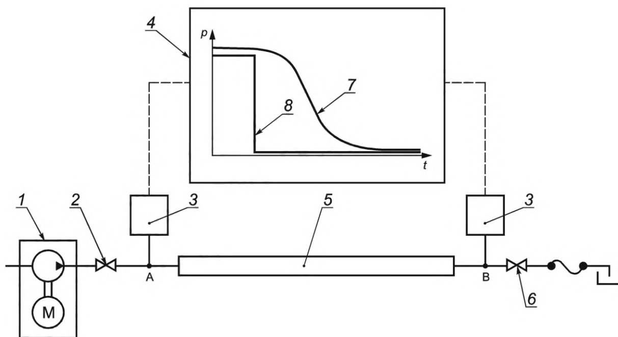
1 — гидравлическая система; 2 — питающий клапан; 3 — преобразователь давления; 4 — ленточный самописец для регистрации зависимости давления от времени; 5 — шлангокабель; 6 — воздушный клапан; 7 — кривая зависимости на конце А; 8 — кривая зависимости на конце В
