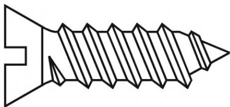
Рисунок 1а — Пример самонарезающего формующего винта
