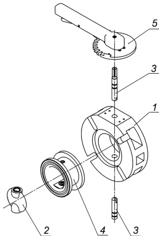
Рисунок 1 — Конструктивные элементы ЗД
