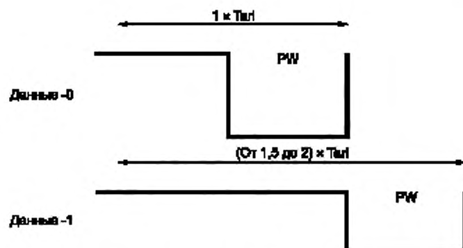
Рисунок 17 — Метод ASK: символы PIE
