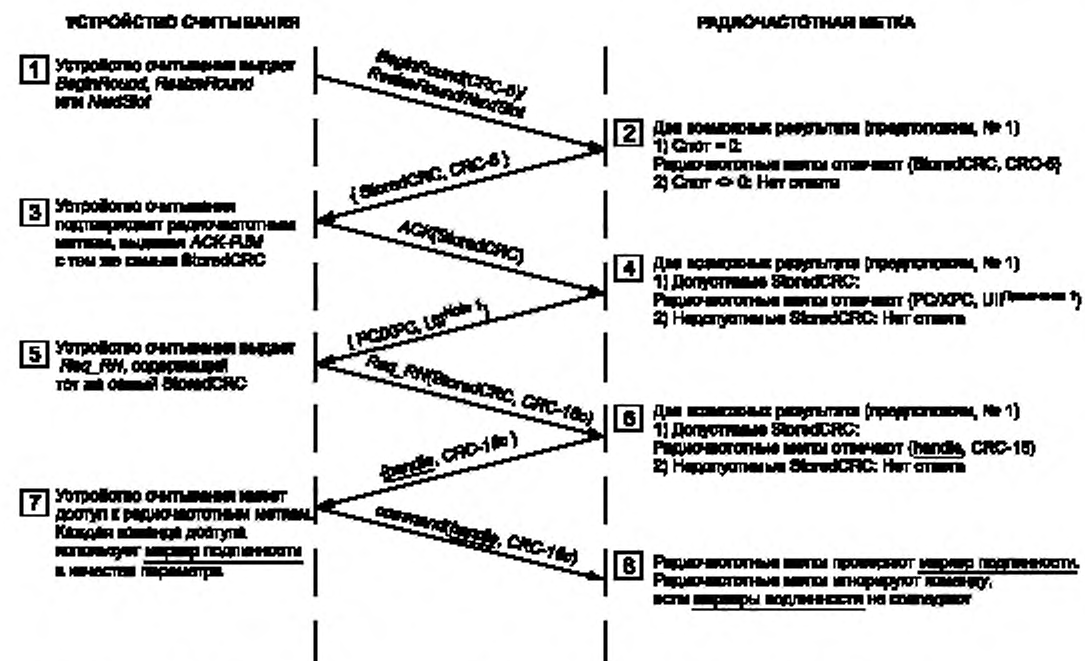
Рисунок H.2 — Метод PJM: Пример инвентаризации и доступа к радиочастотной метке
