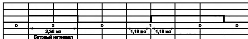
Рисунок 4 — MFM кодирование команды и временные диаграммы двоичной последовательности 000100
