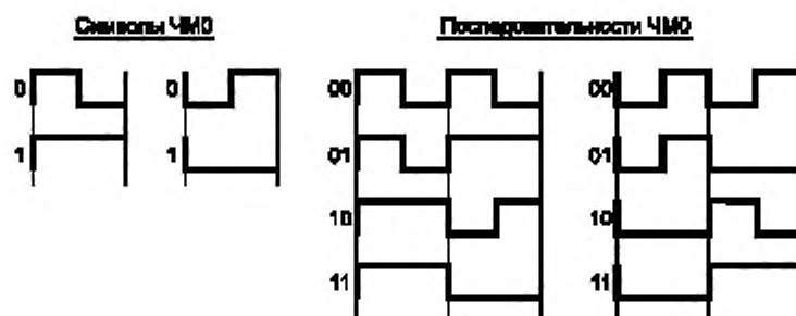
Рисунок 26 — Метод ASK: FM0 символы и последовательности
