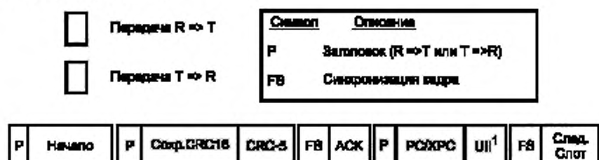
Рисунок 45 — Ответ одной радиочастотной метки
