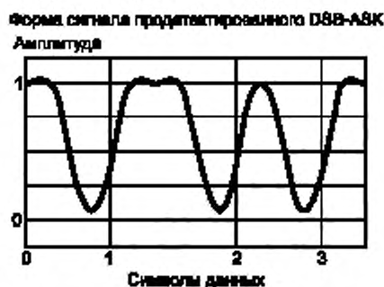
Рисунок J.1 — Модуляция в канале связи «УСО-радиочастотная метка»
