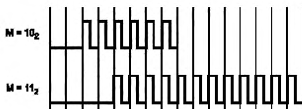
Рисунок 32 — Метод ASK: Символ EOF завершающий передачу поднесущей
