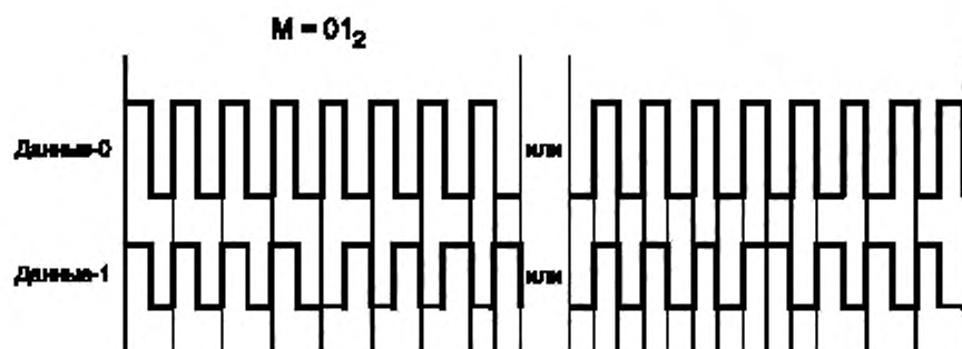
Рисунок 34 — Метод ASK: Последовательность кода Миллера на поднесущей
