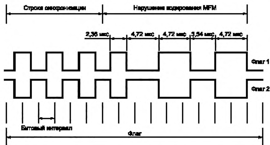
Рисунок 16 — Кодирование и разбиение по времени (согласование по времени) для двух возможных флагов команды в режиме 1 из 4
