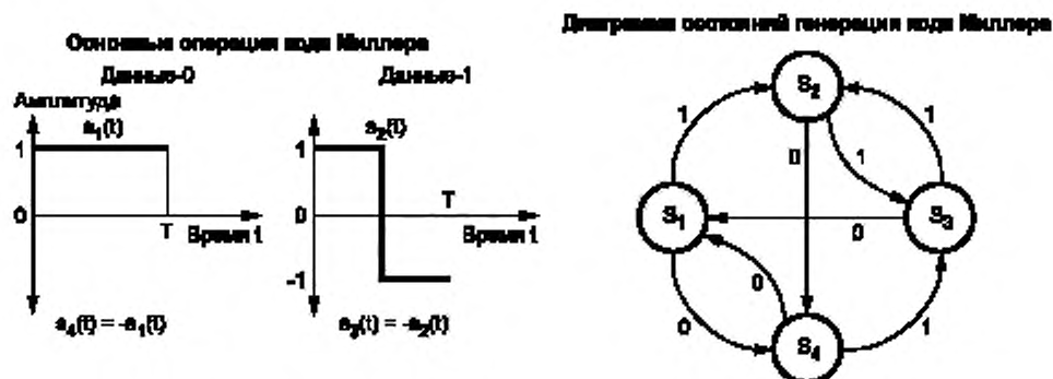
Рисунок 33 — Метод ASK: Основные операции кода Миллера и диаграмма состояний генерации кода
