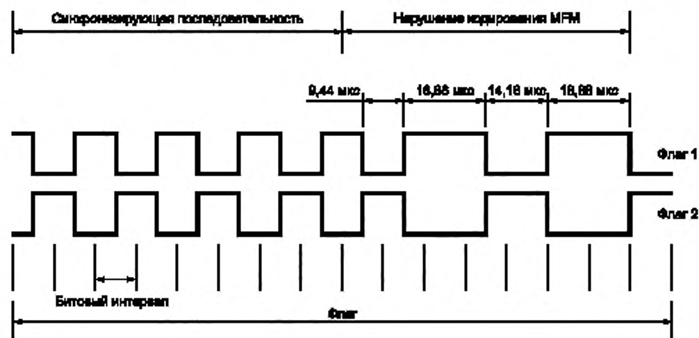
Рисунок 8 — MFM кодирование и временные диаграммы для двух возможных флагов ответа
