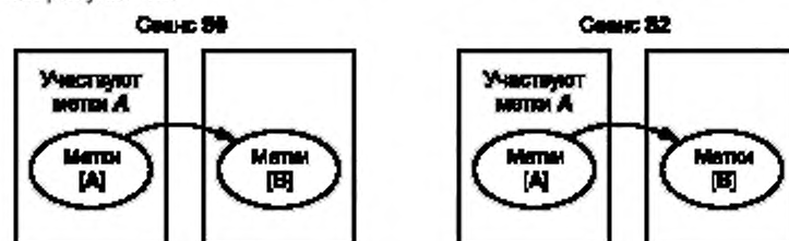
Рисунок 42 — Диаграмма сеансов
