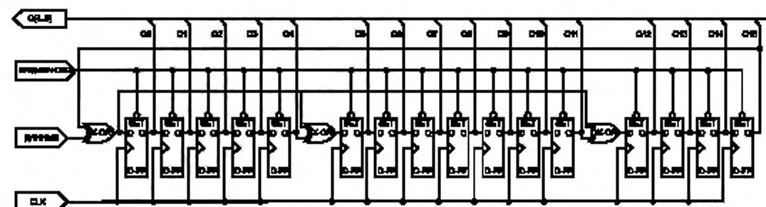
Рисунок 1.2 — Пример схемы кода CRC-16с
