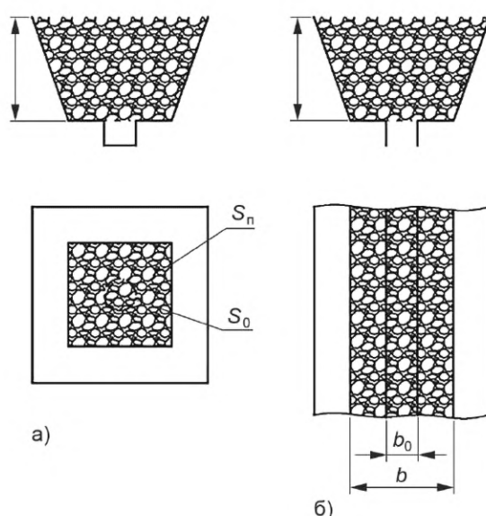
Рисунок 15.15 — Обрушение в форме усеченной пирамиды ( S_0 < S_n )
