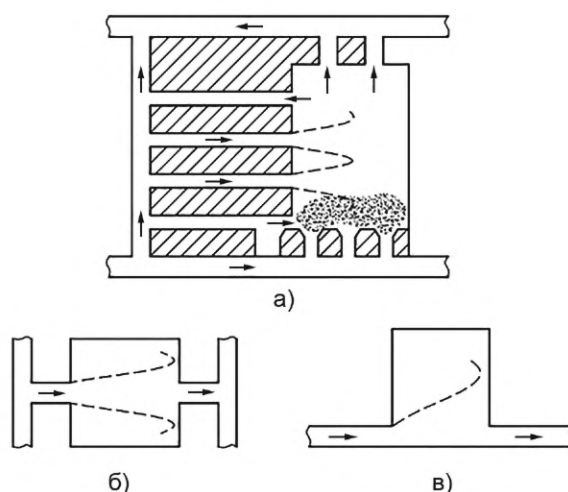
Рисунок 15.1 — Типы камерообразных выработок
