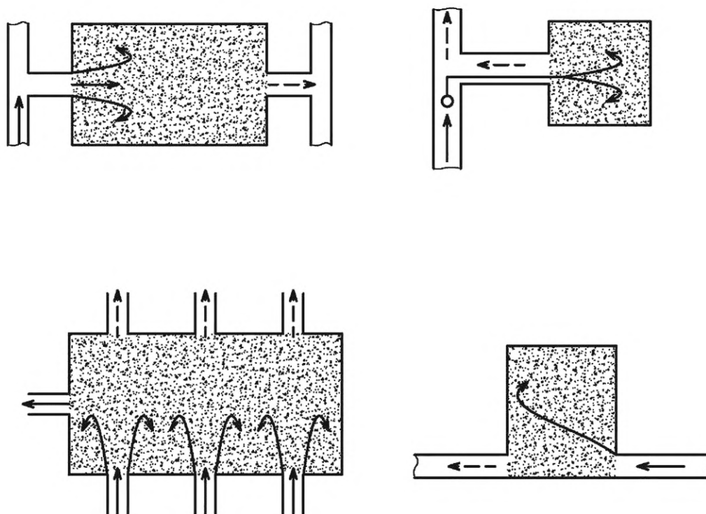
Рисунок 15.6 — Схемы проветривания выработок свободными струями
