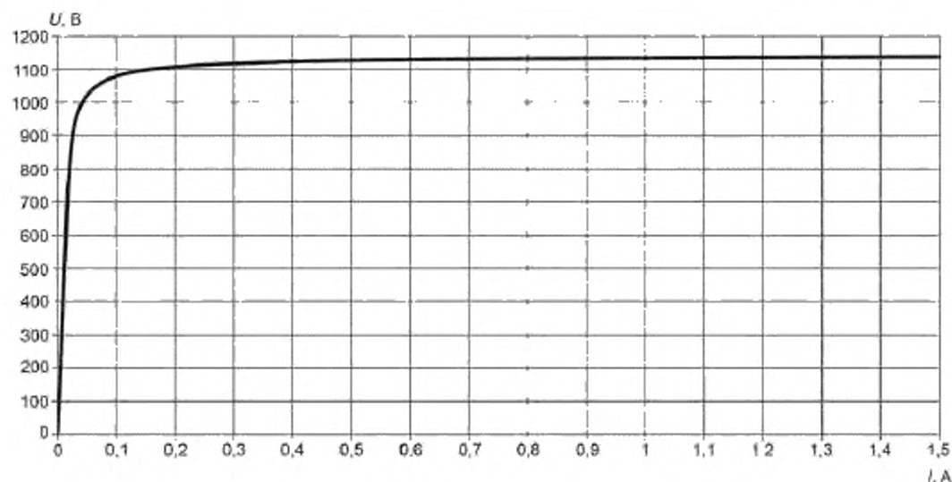
Рисунок В.3 — Вольтамперная характеристика ТТ SAS 550/5G 2000/1
