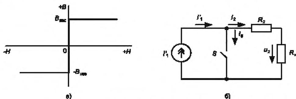
Рисунок 7.2 — Идеальная прямоугольная характеристика ПХН, а), и схема замещения ТТ с ПХН, б), при активном характере сопротивления ветви вторичного тока
