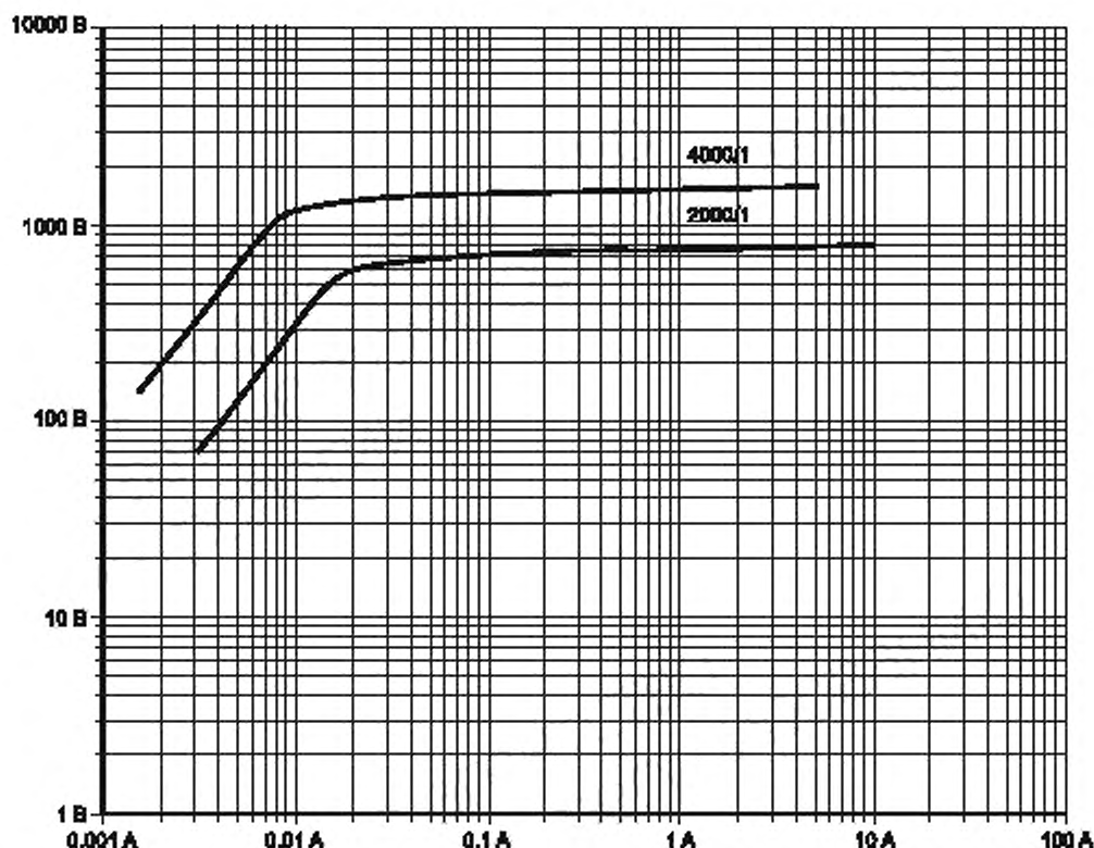
Рисунок В.5 — Вольтамперная характеристика ТТ JK ELK СВ3—780 с n_{\text{ном}} 4000/1 (верхняя кривая) и 2000/1 (нижняя кривая)
