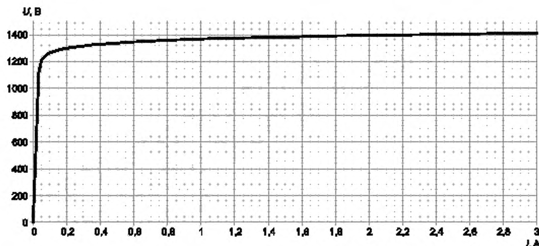
Рисунок В.4 — Вольтамперная характеристика ТТ ТФ3М—500Б—2000/1
