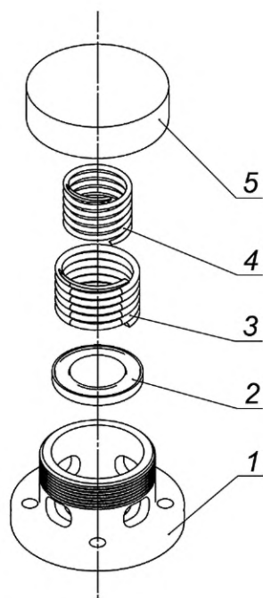
Рисунок 1 — Конструктивные элементы ПК
