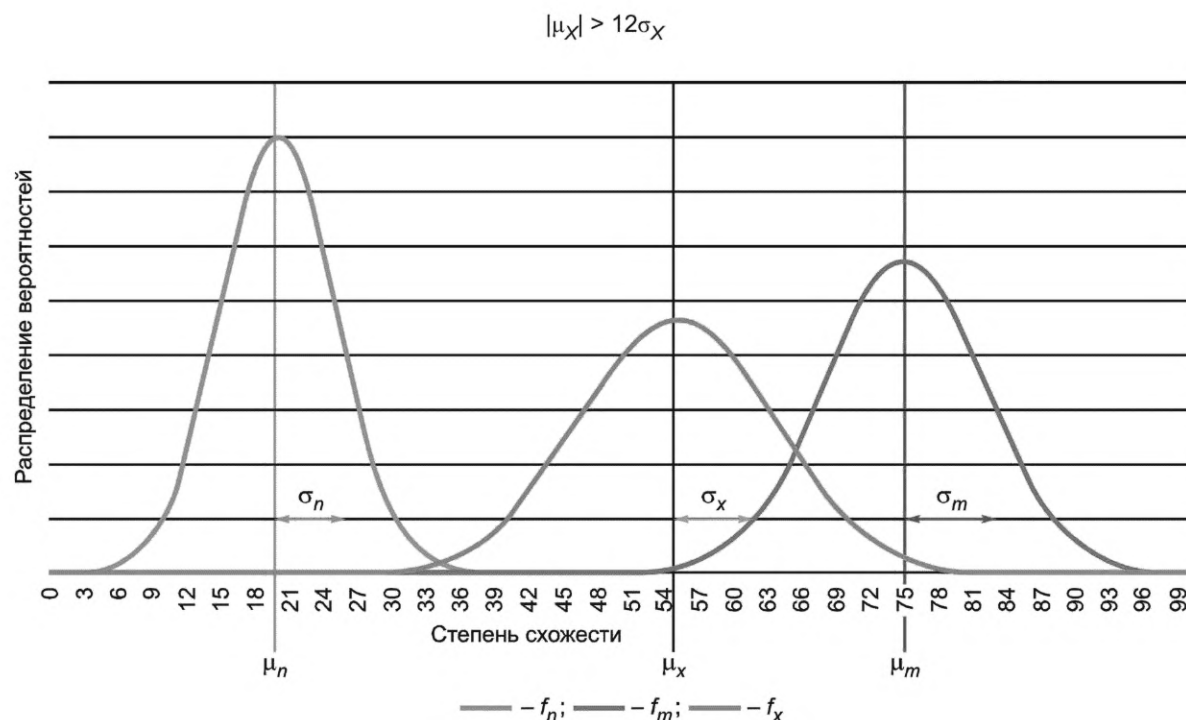
Рисунок D.22 — Распределение различий степеней схожести парных и непарных биометрических образцов
