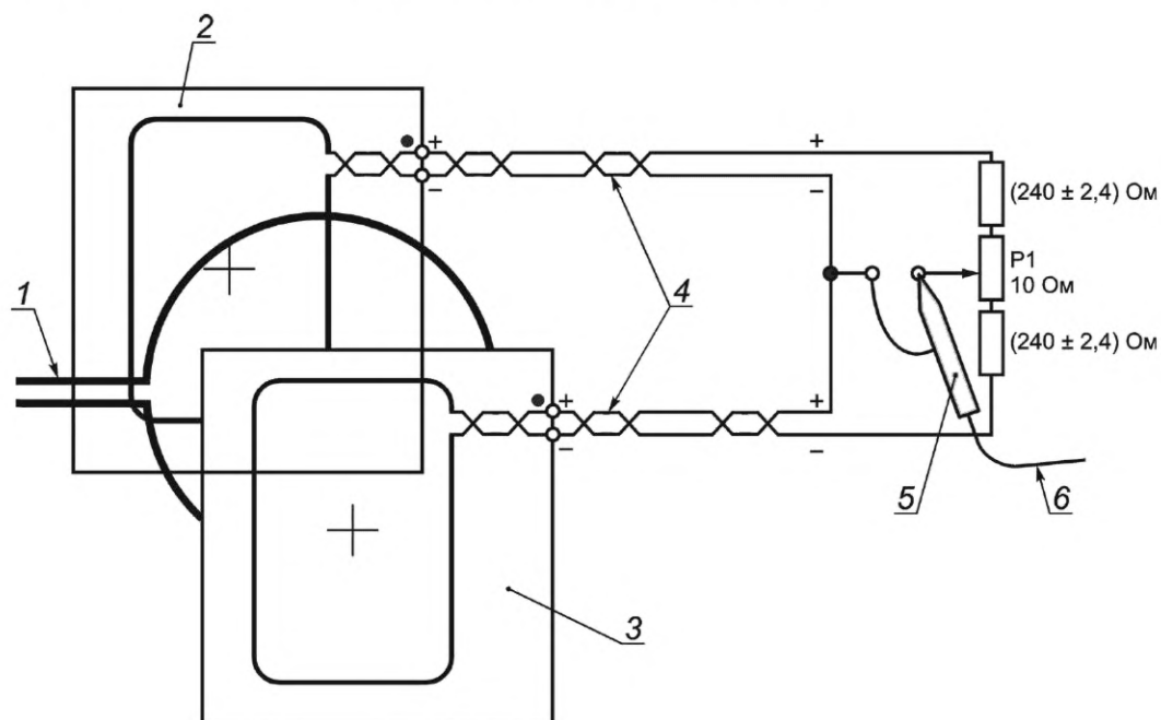
1 — антенна терминального оборудования VCD; 2 — катушка считывания b ; 3 — катушка считывания a ; 4 — одинаковая длина витков пар менее 150 мм; 5 — зонд; 6 — к осциллографу; P1 — потенциометр
