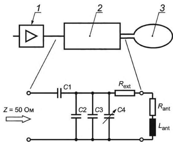
1 — генератор мощности, 50 Ом; 2 — сеть, согласованная по импедансу; 3 — антенная катушка; Z — входной импеданс; R_{ext} — внешнее сопротивление; R_{ant} — сопротивление антенны; L_{ant} — индуктивность антенны; C1, C2, C3, C4 — конденсаторы Рисунок А.3 — Сеть, согласованная по импедансу
