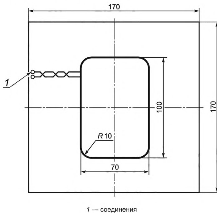
Рисунок С.1 — Компоновка для катушек считывания а и б
