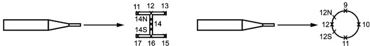
Рисунок Т.3 — Ориентация струи относительно термопар в месте соударения с балкой и с трубой
