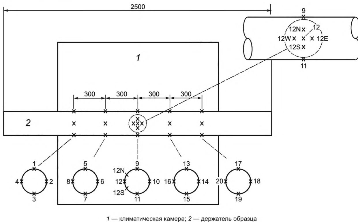
Рисунок Т.2 — Схема мест расположения термопар на трубе
