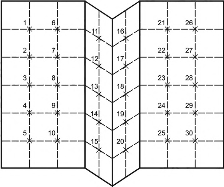
Рисунок Р.1 — Схема мест измерения толщины
