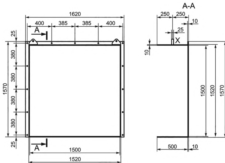
Рисунок Н.1 — Общий вид держателя образца и камеры
