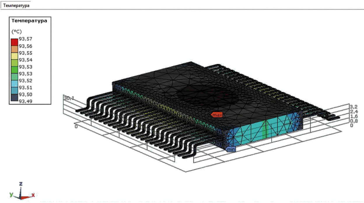
Рисунок А.7 — Температуры во всех точках конструкции блока ЭКБ
