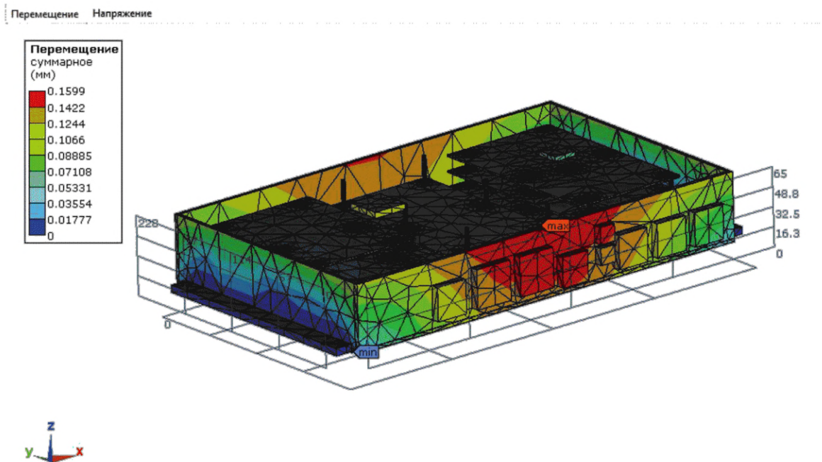
Рисунок А.5 — Суммарные перемещения во всех точках конструкции блока ЭА
