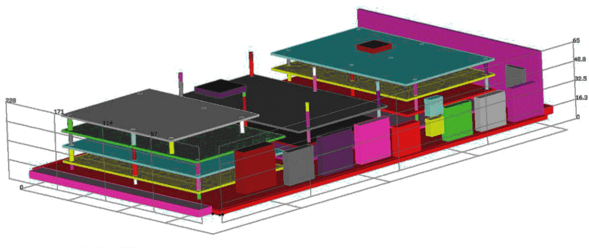
Рисунок А.1 — Конструкция блока ЭА, импортированная из CAD-системы в подсистему АСОНИКА-М-3D
