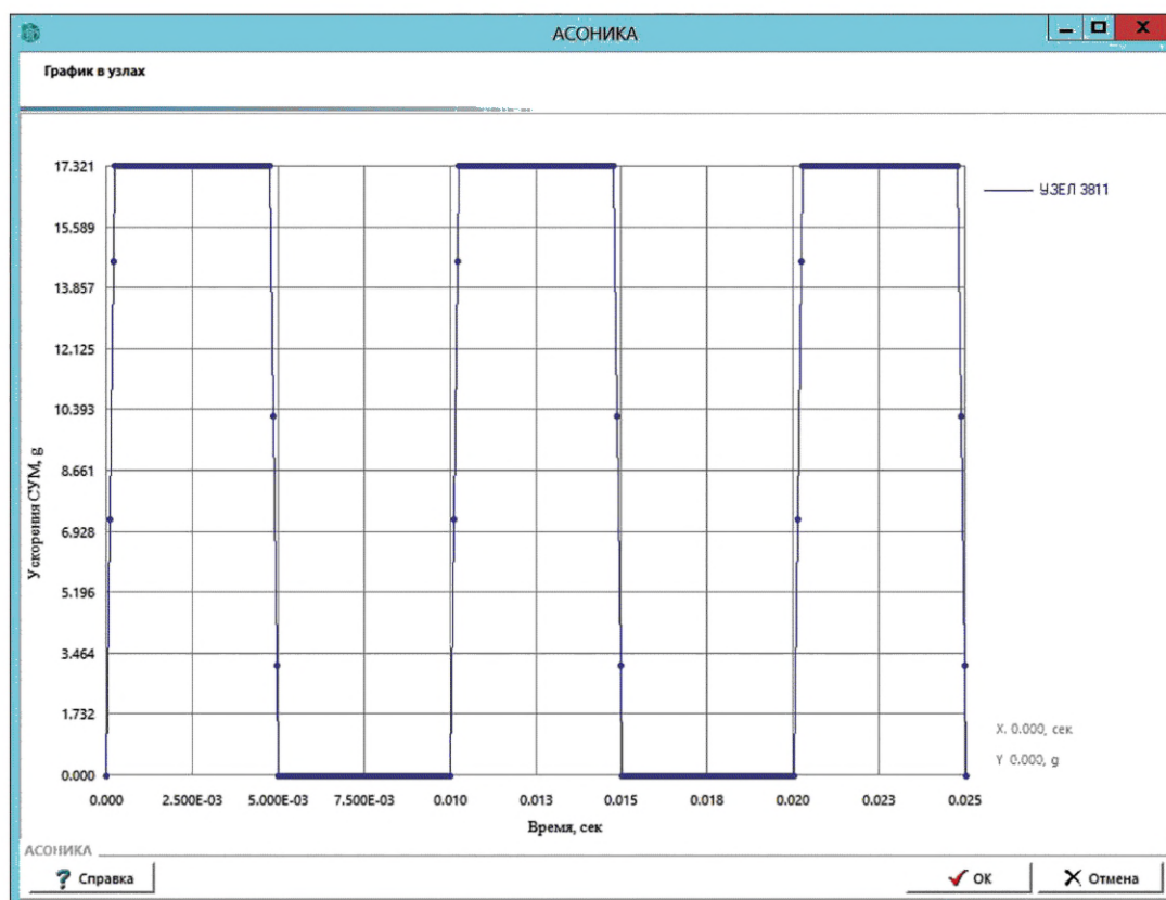
Рисунок А.10 — График зависимости выходного суммарного ускорения многократного механического удара от времени в контрольной точке конструкции ЭКБ
