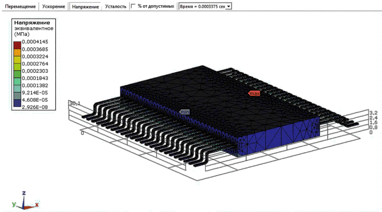
Рисунок А.8 — Эквивалентные механические напряжения во всех точках конструкции ЭКБ при воздействии многократного механического удара в заданный момент времени
