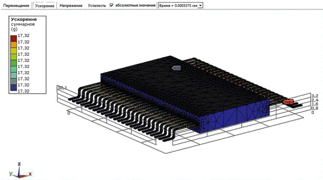
Рисунок А.7 — Суммарные ускорения во всех точках конструкции ЭКБ при воздействии многократного механического удара в заданный момент времени
