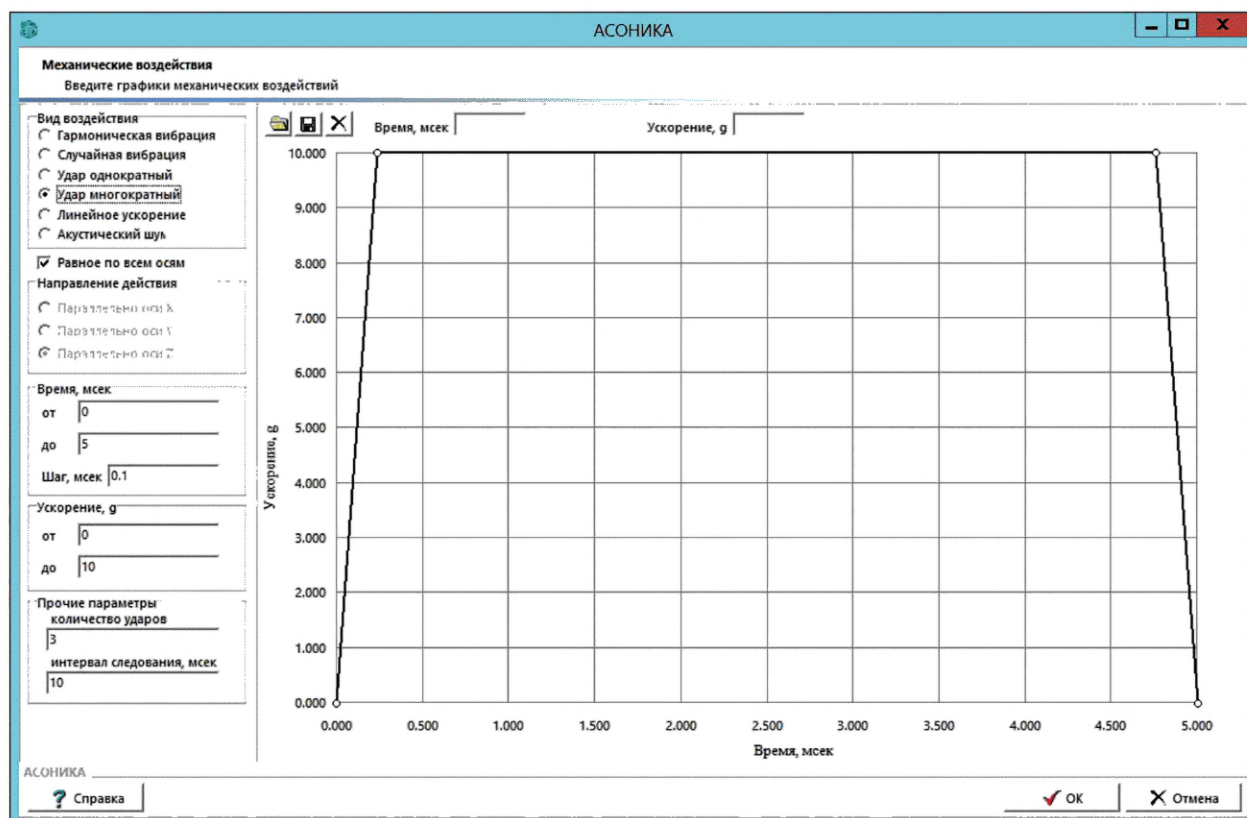
Рисунок А.5 — График зависимости входного суммарного ускорения многократного механического удара от времени
