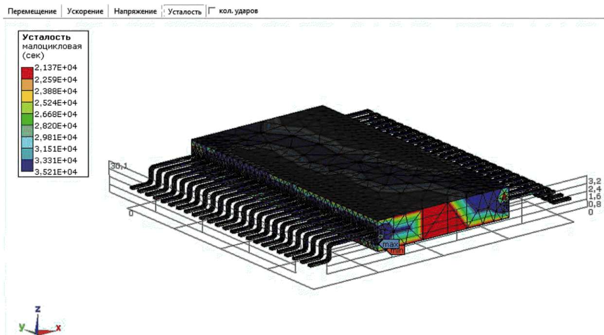
Рисунок А.9 — Время до усталостного разрушения во всех точках конструкции ЭКБ при воздействии многократного механического удара
