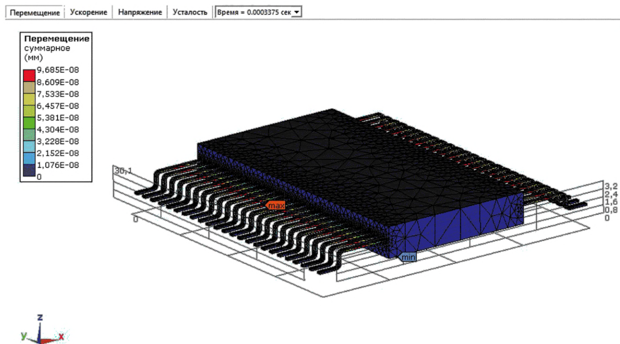
Рисунок А.6 — Суммарные перемещения во всех точках конструкции ЭКБ при воздействии многократного механического удара в заданный момент времени
