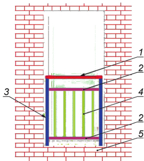
в) Решетчатый защитный экран с комбинированным креплением
