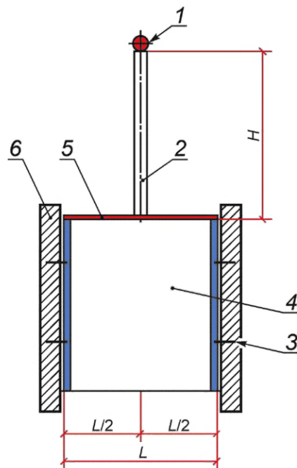
1 — стальной шар диаметром 63,5 мм; 2 — направляющая труба с внутренним диаметром 64 мм; 3 — элементы крепления защитного экрана к каркасу испытательного стенда; 4 — безопасное стекло защитного экрана; 5 — кромочный профиль либо поручень; 6 — каркас испытательного стенда; H — высота направляющей трубы; L — ширина защитного экрана
