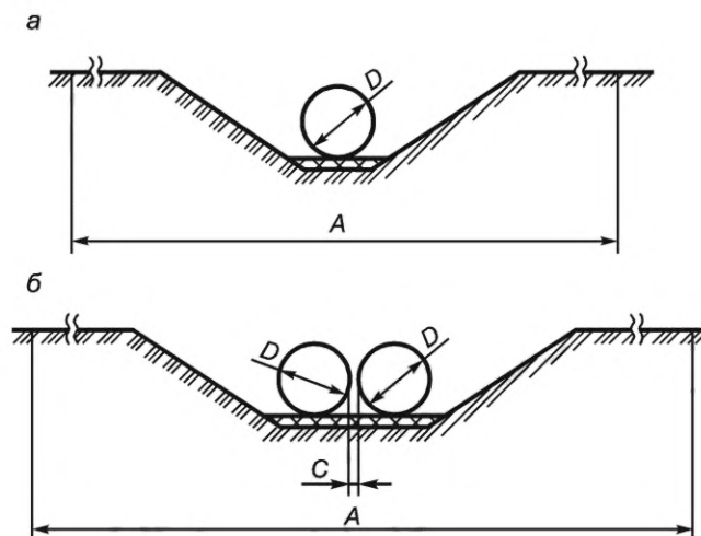
а — укладка трубопровода в одну нитку; б — укладка трубопровода в две нитки; D — диаметр трубопровода, м; A — ширина полосы отвода, м; C — расстояние между наружными диаметрами труб, м
