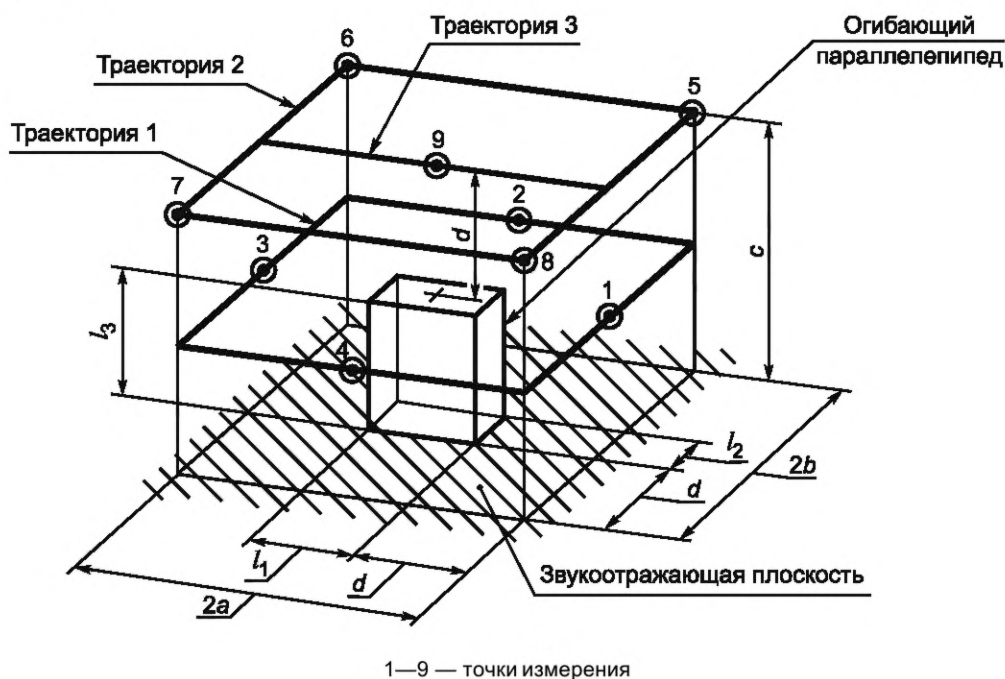
Рисунок 1 — Пример измерительной поверхности и положений (траекторий) микрофонов
