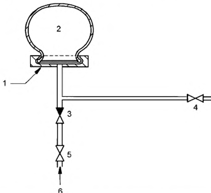
1 – кольцо, фиксирующее диафрагму; 2 – растянутая диафрагма; 3 – не возвратный клапан; 4 – воздушный выпускной клапан; 5 – клапан; 6 – источник подачи воздуха под давлением
