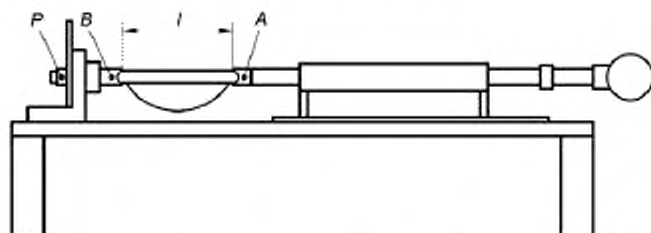
Рисунок F.1 — Оборудование для скручивания диафрагмы
