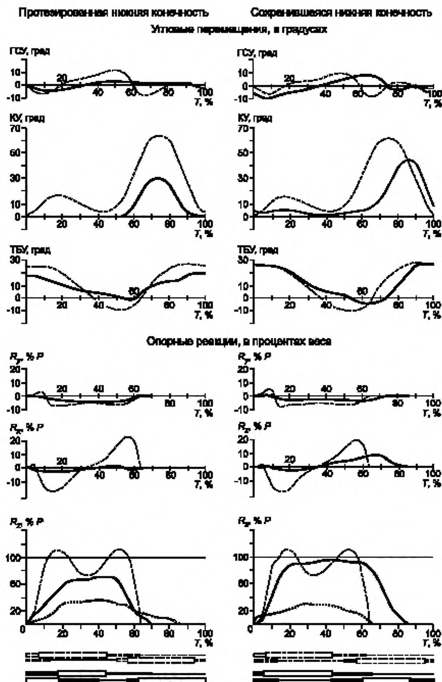
Рисунок А.2 — Графики изменения средних значений угловых перемещений (в суставах нижних конечностей и шарнирах протеза) и составляющих опорной реакции за время двойного шага при ходьбе на протезах бедра мужчин с культей сосудистого генеза (условная норма) и при ходьбе в норме
