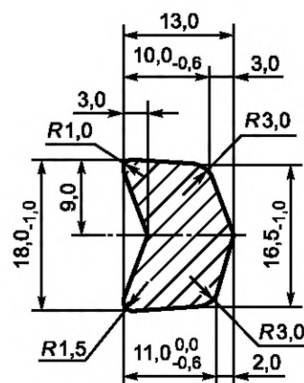
Рисунок А.3 — Бандажное кольцо
