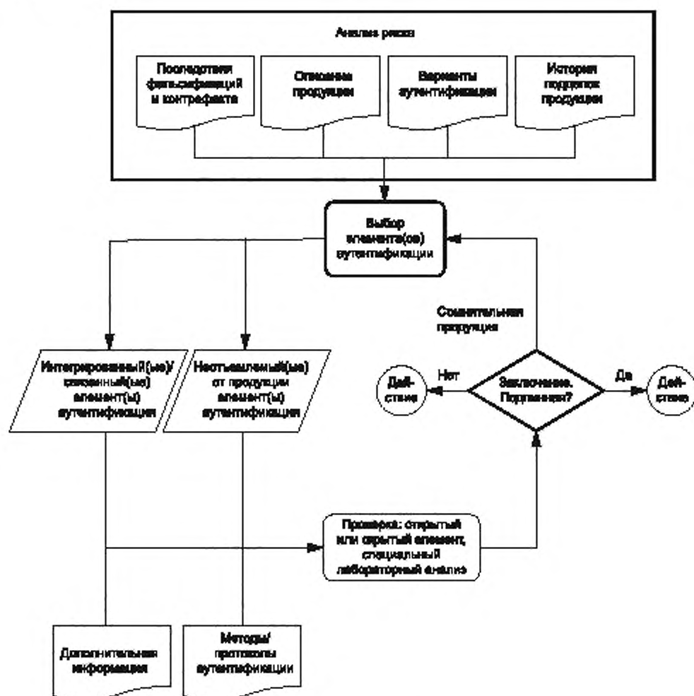
Рисунок 1 — Функциональная схема типового средства аутентификации
