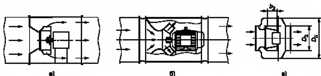
Рисунок 4 — Канальные круглые вентиляторы с цилиндрическим корпусом с радиальным (а) и диагональным (б) рабочим колесом, с торообразным корпусом с радиальным рабочим колесом (в)
