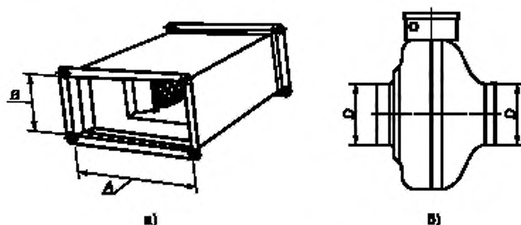
Рисунок 5 — Канальные вентиляторы с прямоугольными (а) и круглыми (б) входными и выходными фланцами
