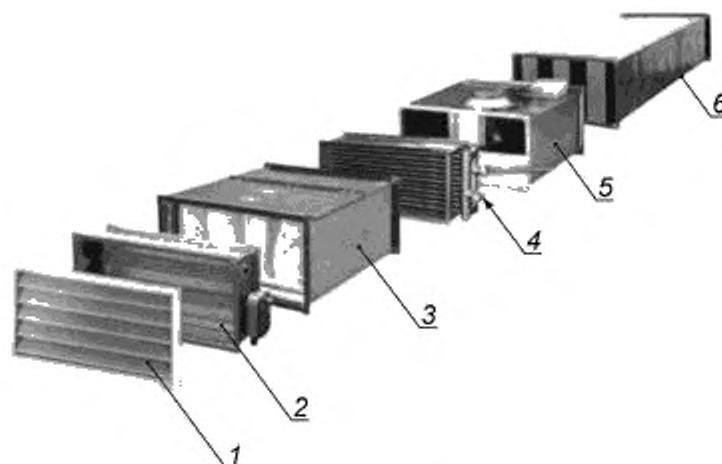
1 — уличная решетка; 2 — клапан с электроприводом; 3 — фильтр; 4 — водяной нагреватель; 5 — канальный вентилятор; 6 — шумоглушитель
