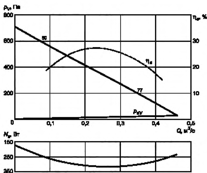
Рисунок А.1 — Аэродинамическая характеристика нерегулируемого канального вентилятора с максимальным значением полного КПД 27,2 %. KEG = 27
