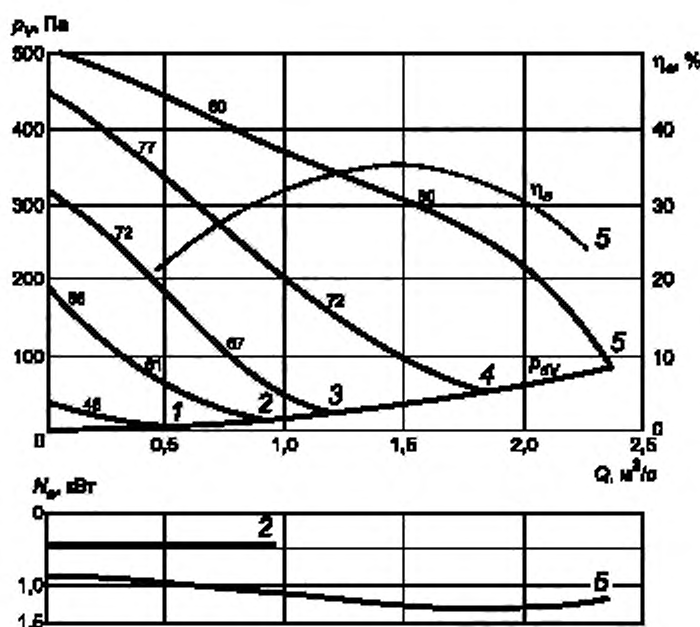
Рисунок А.2 — Аэродинамическая характеристика регулируемого канального вентилятора с максимальным значением полного КПД 35,2 %, KEG = 35
