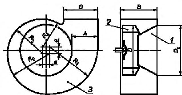
1 — входной коллектор, 2 — рабочее колесо, 3 — спиральный корпус
