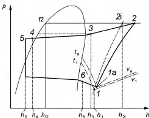
b — Диаграмма давление — энтальпия
