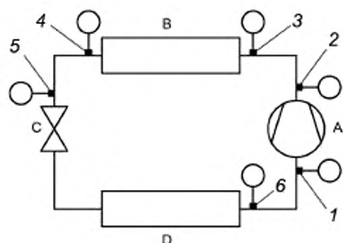
а — Схема цикла
