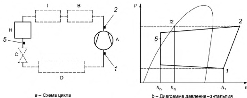
1 — хладагент на входе в компрессор для заданных условий испытания; 2 — хладагент на выходе из компрессора; 5 — жидкий хладагент на входе в расширительное устройство; А — компрессор; В — конденсатор; С — расширительное устройство; D — испаритель; Н — жидкостный ресивер; I — переохладитель
