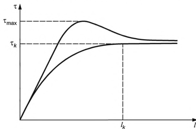
Рисунок Г.1 — График l = f(\tau)
