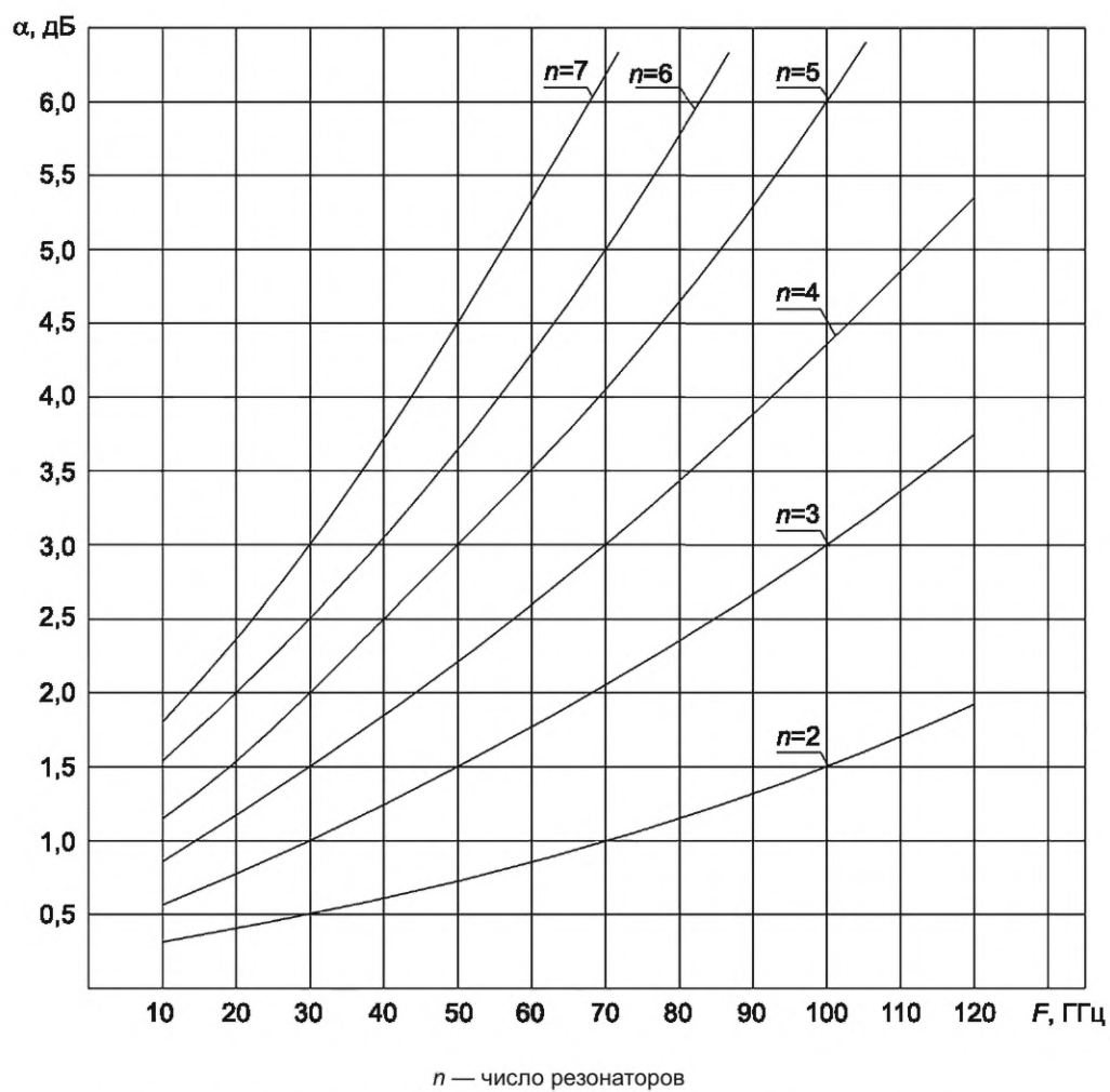
Рисунок 10 — Частотная зависимость минимального затухания \alpha ППФ СВЧ из керамического материала IIIж-4 (KCBH — 2,0)
