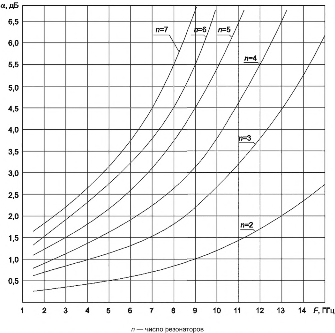
Рисунок 5 — Частотная зависимость минимального затухания \alpha ППФ СВЧ из керамического материала IIIж-4 (KCBH — 2,0)
