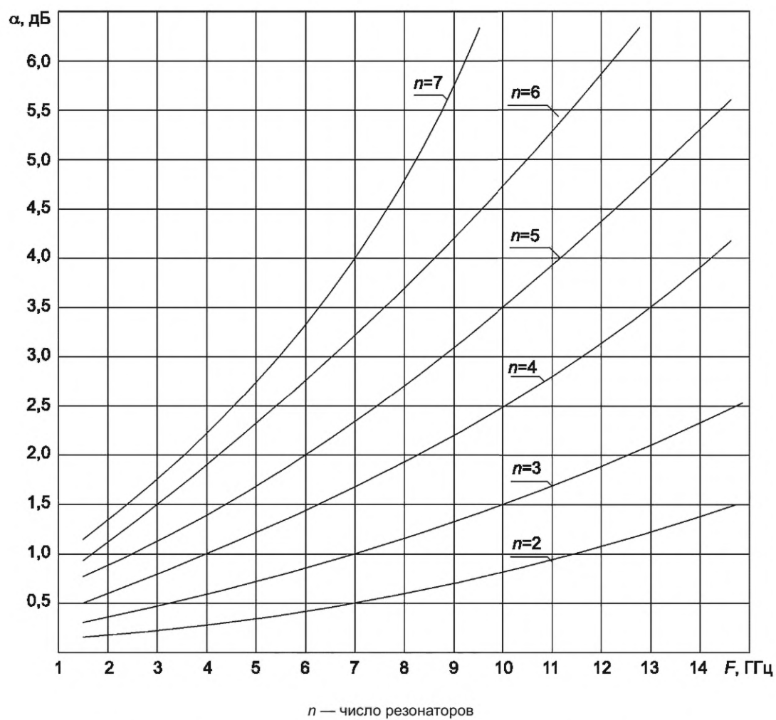
Рисунок 3 — Частотная зависимость минимального затухания \alpha ППФ СВЧ из керамического материала IIIж-4 (KCBH — 1,3)
