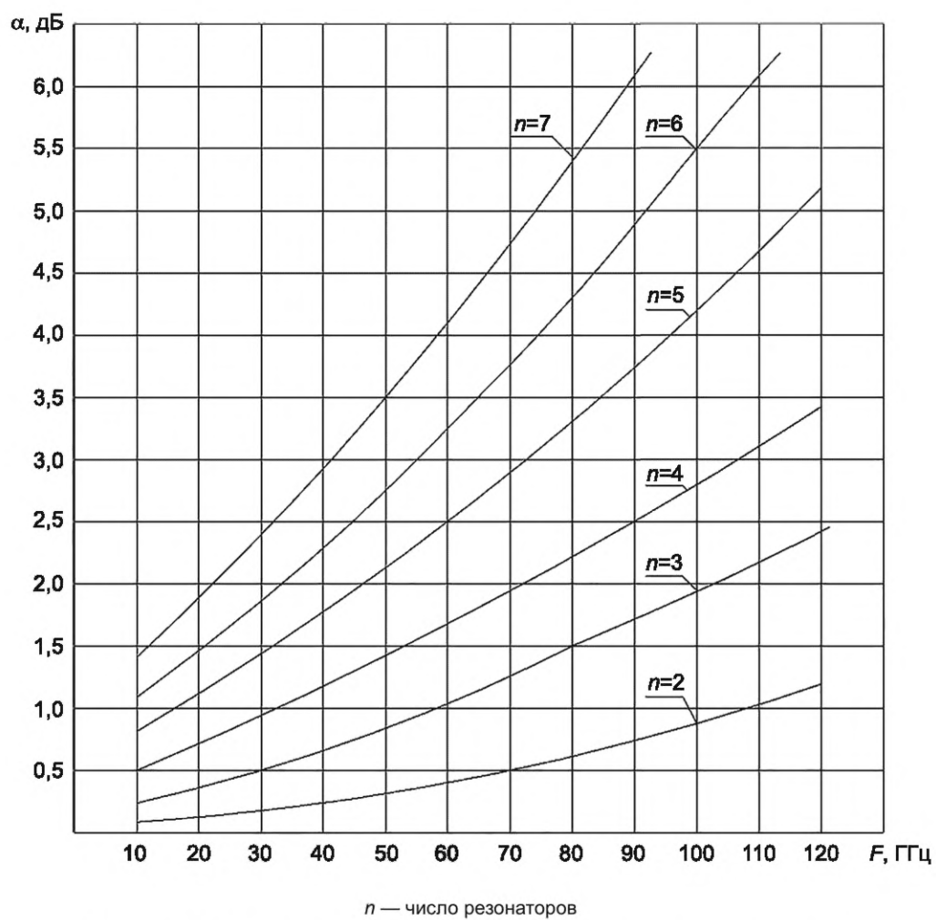
Рисунок 6 — Частотная зависимость минимального затухания \alpha ППФ СВЧ из керамического материала IIIж-4 (KCBH — 1,15)
