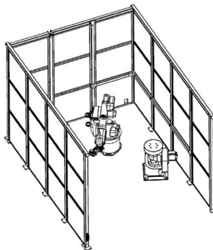
б) Стационарное периферийное ограждение
