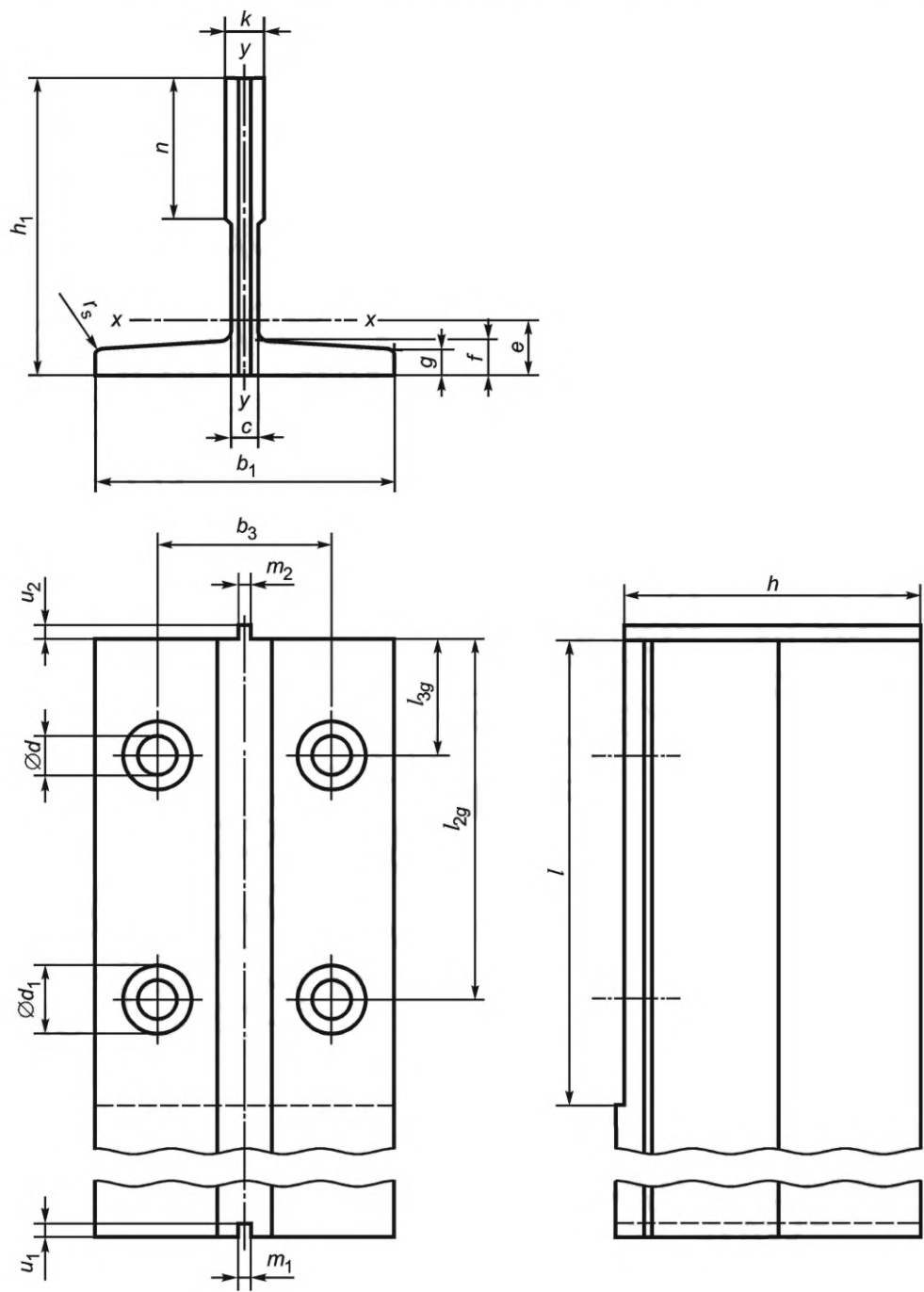
Рисунок 3 — Механически обработанная направляющая
