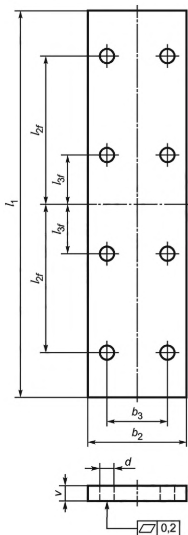
Рисунок 6 — Стыковая планка
