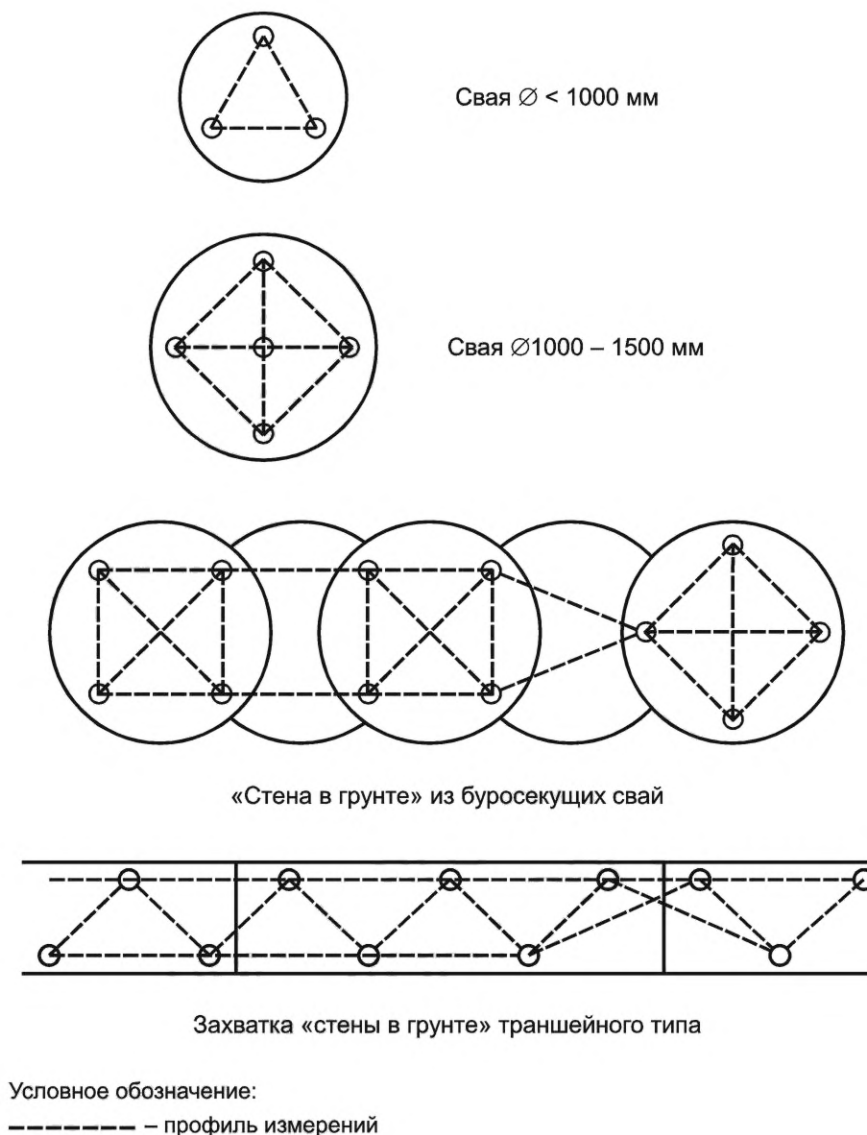
Рисунок 6.1 — Рекомендованная схема расположения труб доступа и профилей измерений
