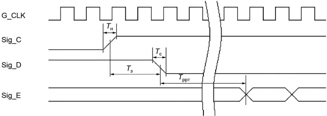
Рисунок 2 — Пример оформления временной диаграммы и описания временных характеристик СФ-блока
