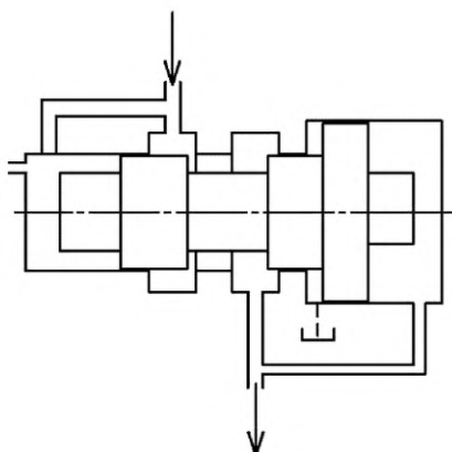
Рисунок 36 — Предохранительный гидроклапан
