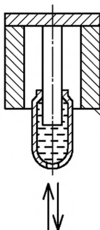
Рисунок 48 — Грузовой гидроаккумулятор
