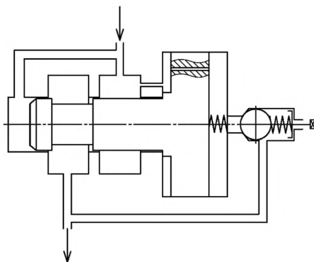
Рисунок 31 — Гидроклапан непрямого действия
