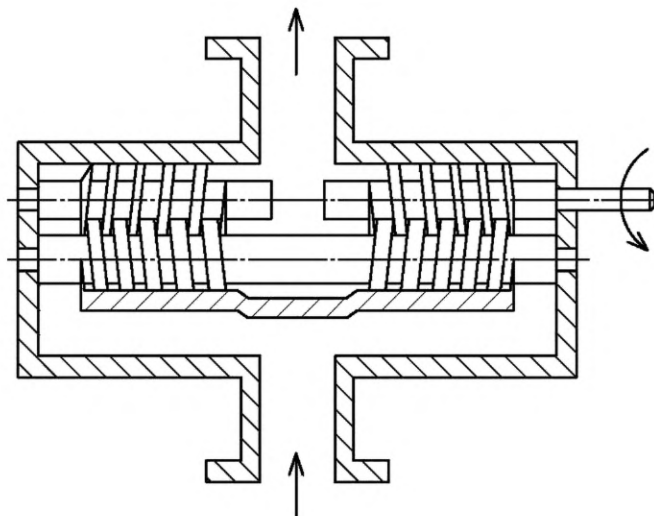
Рисунок 15 — Винтовой гидромотор
