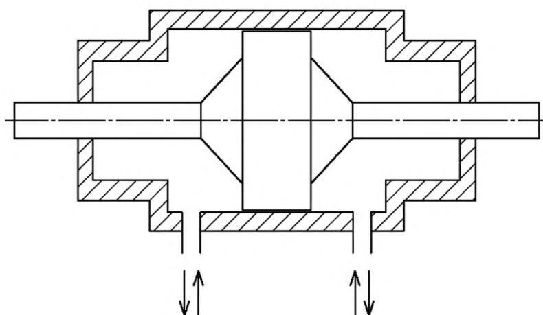
Рисунок 10 — Гидроцилиндр с торможением
