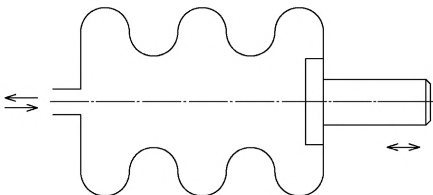
Рисунок 8 — Сильфонный гидроцилиндр
