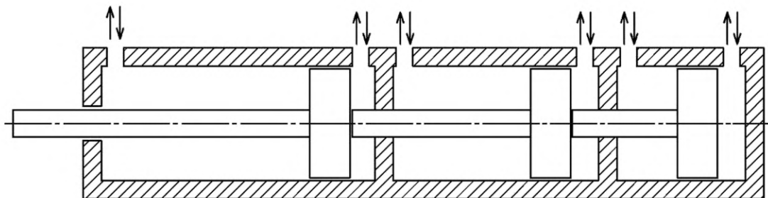
Рисунок 4 — Многопозиционный гидроцилиндр
