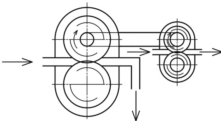
Рисунок 26 — Вращательный гидропреобразователь
