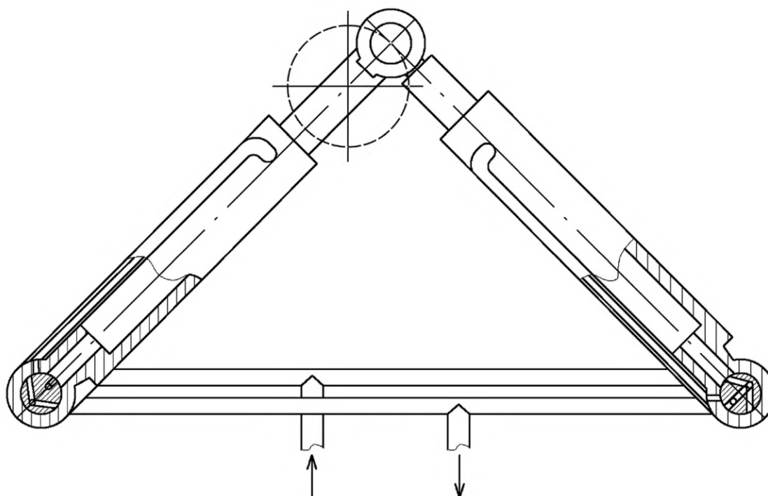
Рисунок 22 — Кривошипный гидромотор
