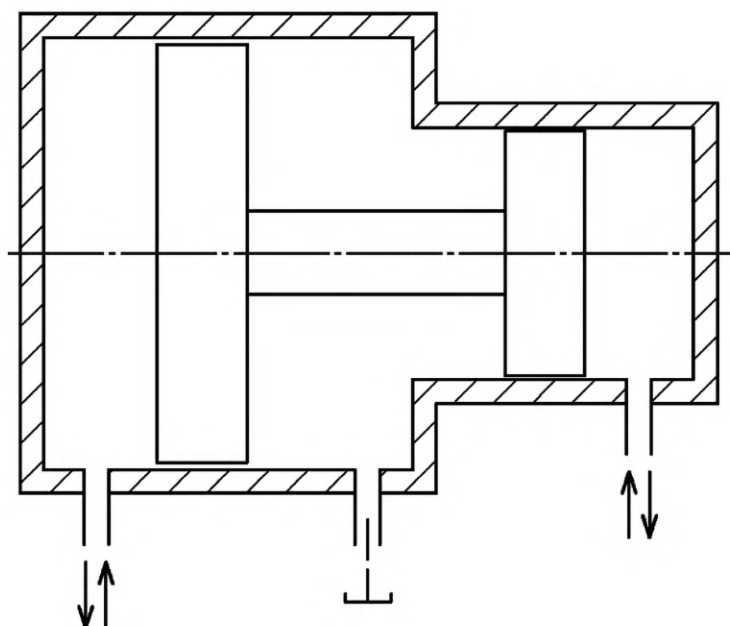
Рисунок 25 — Поступательный гидропреобразователь
