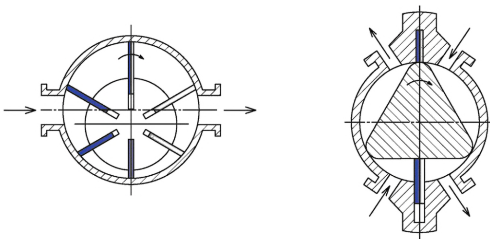
Рисунок 18 — Пластинчатый гидромотор
