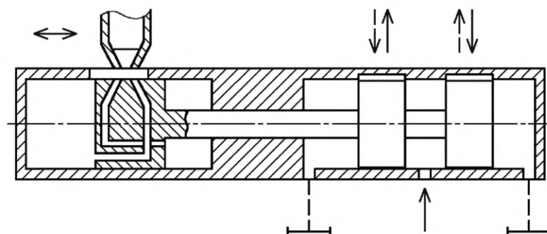
Рисунок 53 — Гидроусилитель
