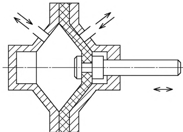
Рисунок 7 — Мембранный гидроцилиндр
