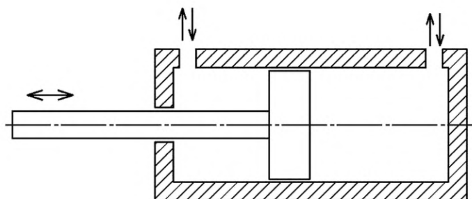
Рисунок 5 — Поршневой гидроцилиндр
