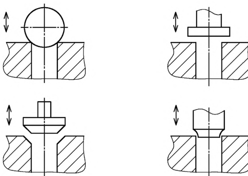
Рисунок 29 — Клапанный гидроаппарат
