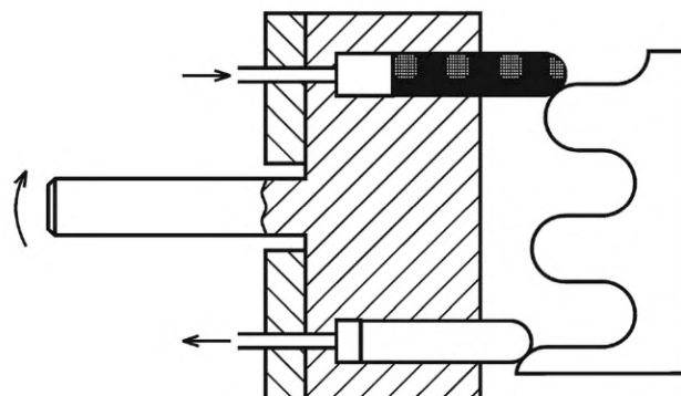
Рисунок 21 — Гидромотор с профильным диском
