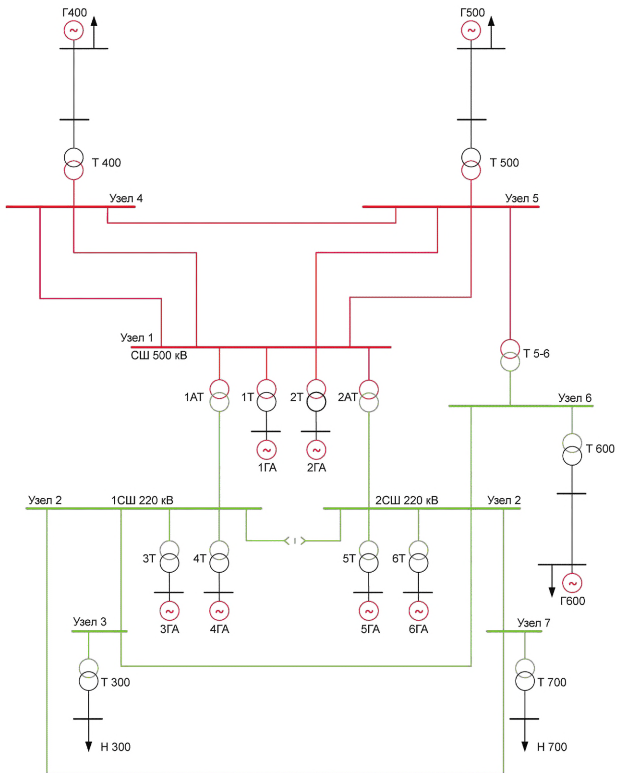
Рисунок А.1 — Общая схема тестовой модели энергосистемы
