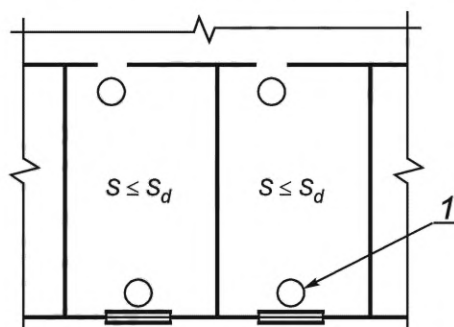
1 — ороситель; S — площадь сдерживания пожара; S_d — допустимая площадь сдерживания пожара
