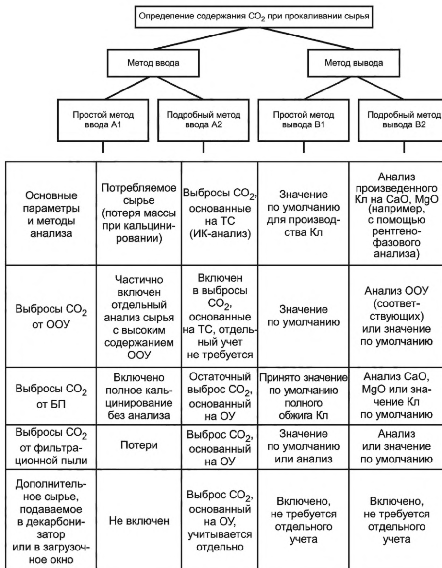
Рисунок 5 — Обзор методов определения выбросов CO 2 при декарбонизации/кальцинировании сыра
