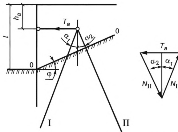
Рисунок 4 — Схема к расчету анкерных козловых опор
