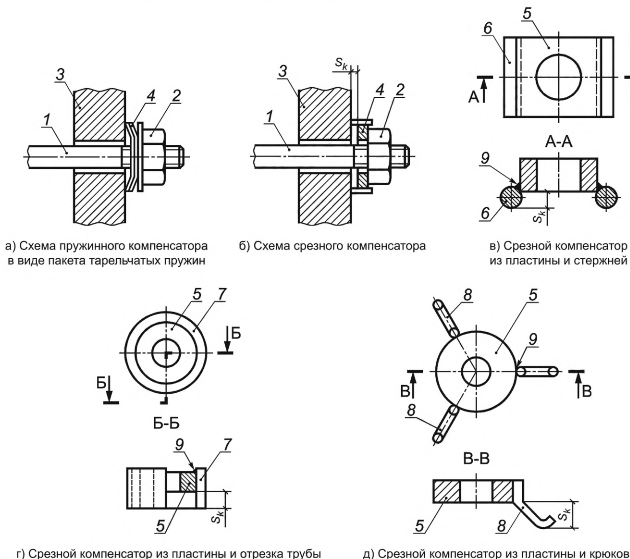
Рисунок 5 — Конструкции компенсаторов в узлах соединения с анкерной плитой или с лицевым элементом
