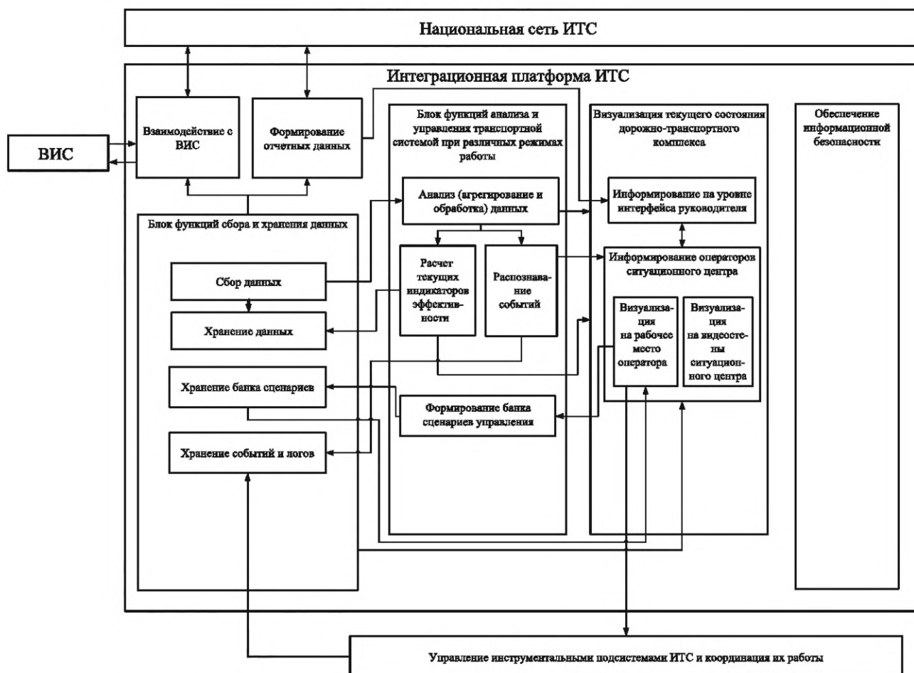
Рисунок А.1 — Общий вид функциональной архитектуры интеграционной платформы первого технологического уровня
