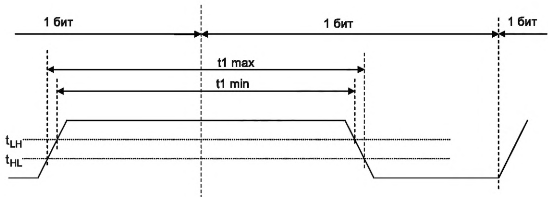
Рисунок 71 — Маска цифрового приема 2
