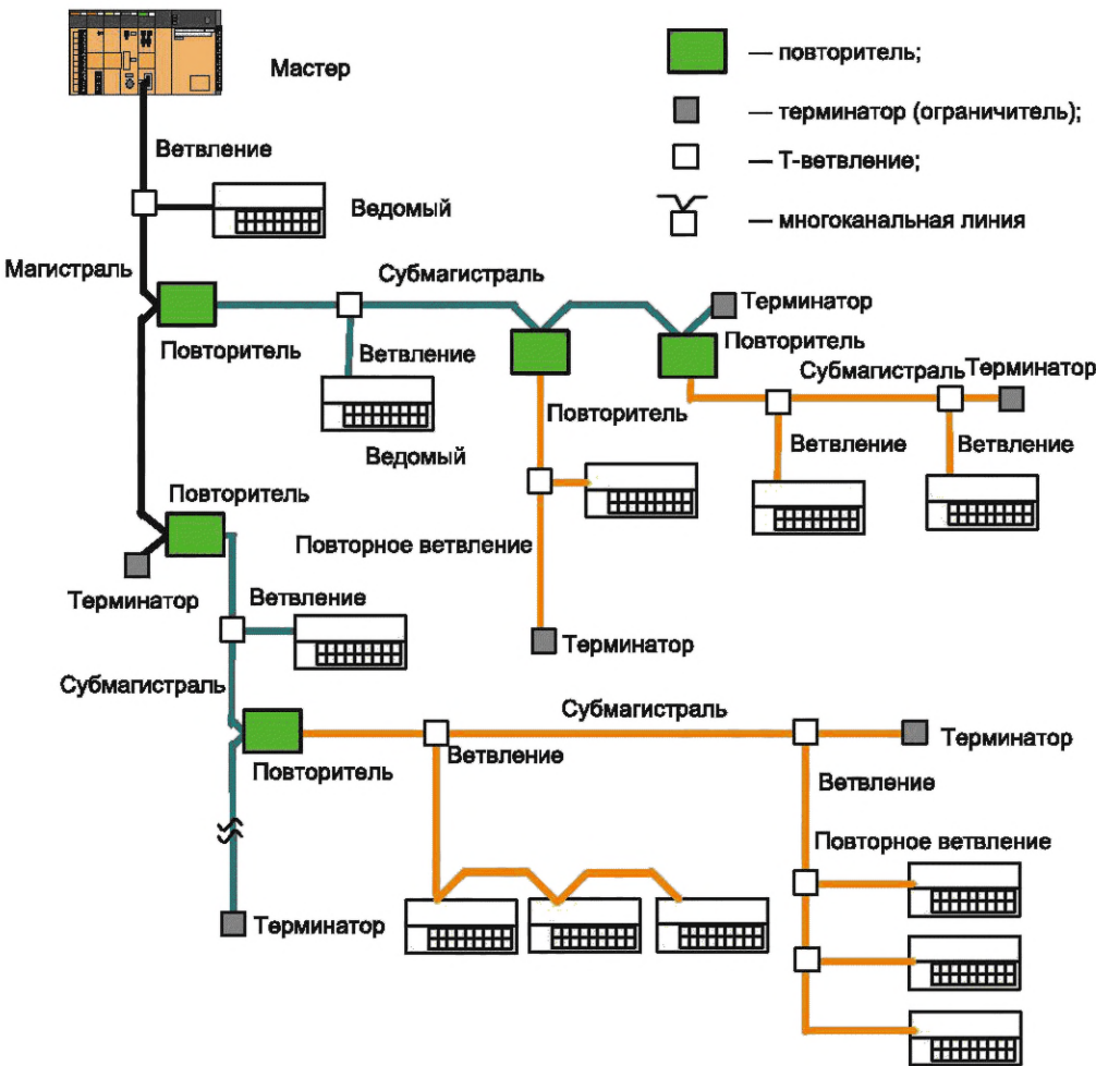
Рисунок 83 — Топология среды передачи данных
