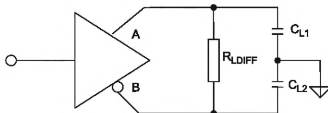
Рисунок 78 — Схема измерения задержки распространения
