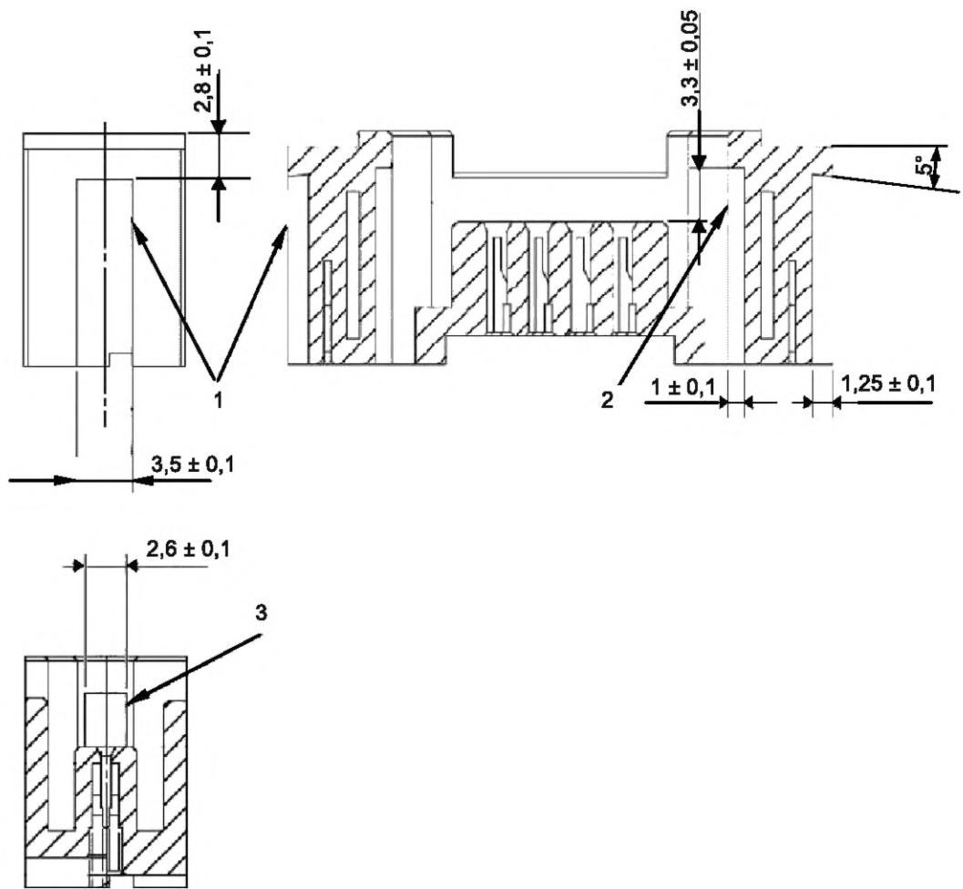
1 — внешние фиксаторы; 2 — внутренние крючки; 3 — внутренние крючки
