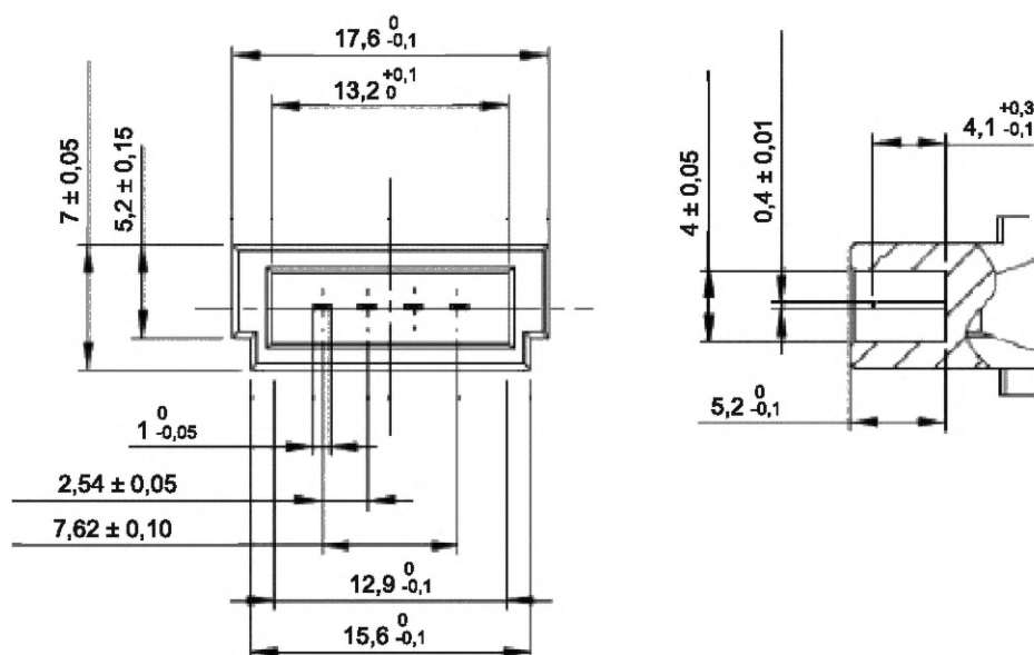
Рисунок 101 — Присоединительные размеры штекерного соединителя
