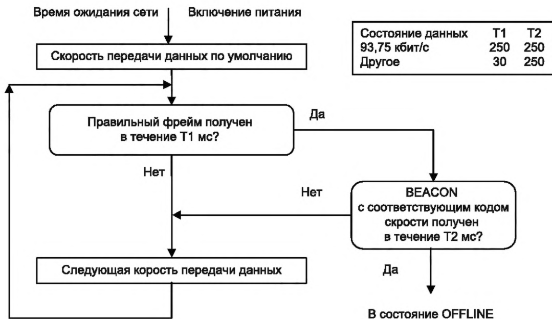
Рисунок 51 — Диаграмма определения скорости передачи данных
