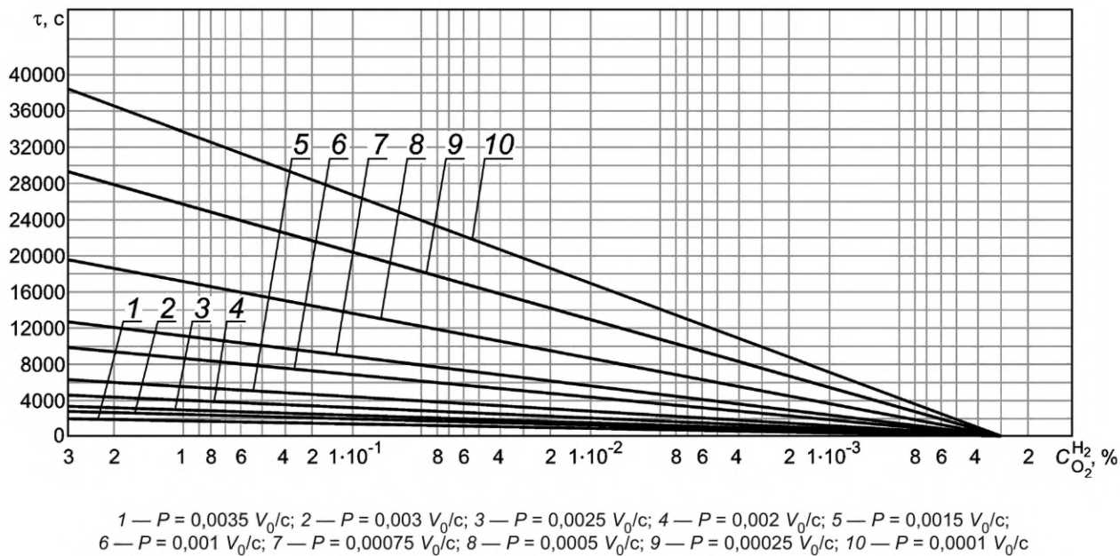
Рисунок В.3 — Ориентировочное время продувки, необходимое для снижения концентрации кислорода от начальной 3,0 \cdot 10^{-4} \% при различных расходах газа. Расход газа в долях объема резервуара в с, а суммарный расход в объемах резервуара
