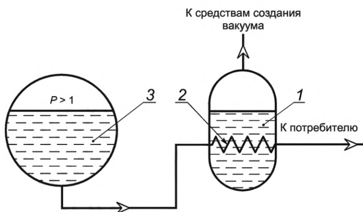
Рисунок Ж.1 — Прямое вакуумирование
