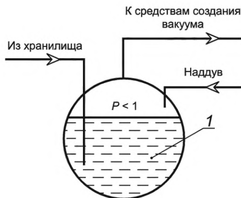
Рисунок Ж.1 — Прямое вакуумирование
