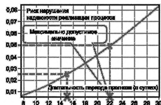
Рисунок Г.8 — Зависимость риска нарушения надежности реализации процесса (без учета требований по защите информации) от длительности периода прогноза
