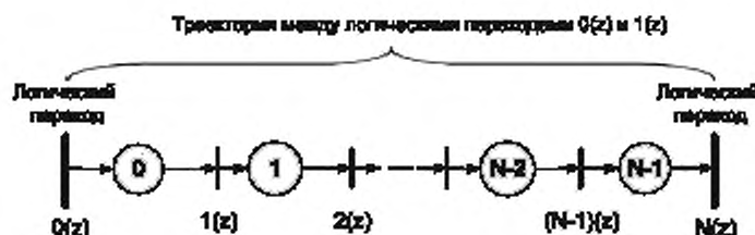
Рисунок Д.9 — Траектория перемещения подпроцесса по сети Петри—Маркова по одной из траекторий между двумя логическими переходами
