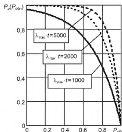
Рисунок Д.1 — Зависимость вероятности реализации компьютерной атаки «SYN-flooding» от вероятности ее обнаружения и блокирования при J_{пред} = 300
