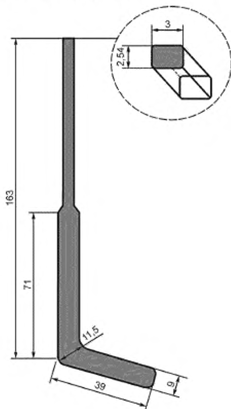
Рисунок 2 — Клюшка вратаря
