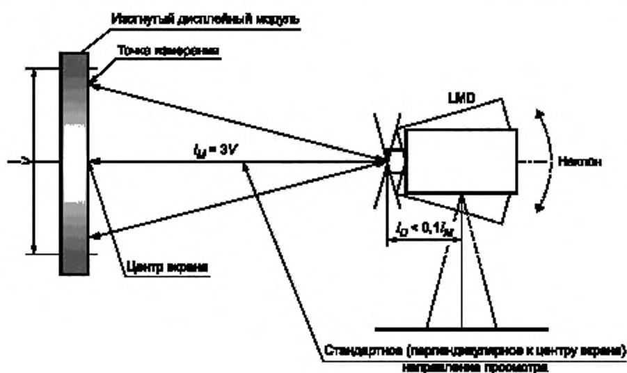
Рисунок 3 — Геометрия измерений в вертикальной точке наиболее благоприятного просмотра (вид сверху)
