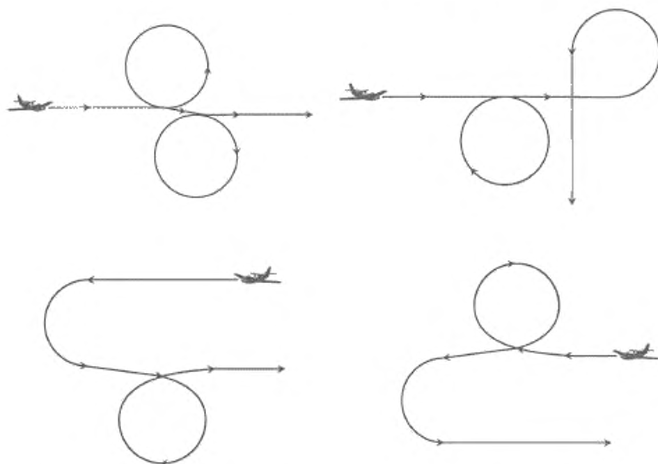
Рисунок В.1 — Варианты траекторий полета при выполнении процедуры инициализации бортового инерциального измерительного устройства
