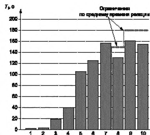
Рисунок Г.6 — Среднее время реакции по 10 типам информации
