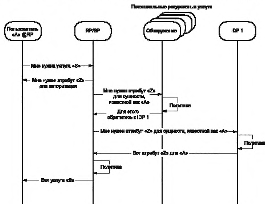
Рисунок А.4 — Пример основного диалога процесса обнаружения в объединении
