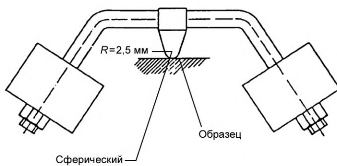
Рисунок 15 — Аппарат для испытания на твердость давлением шарика (9.13.2)
