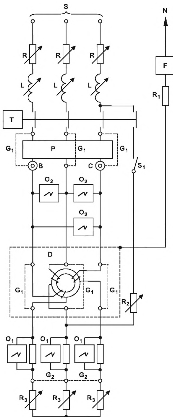
Рисунок 6 — Испытательная цепь для проверки координации с устройством SCPD прибора RCM с тремя путями тока в трехфазной цепи (9.11)
