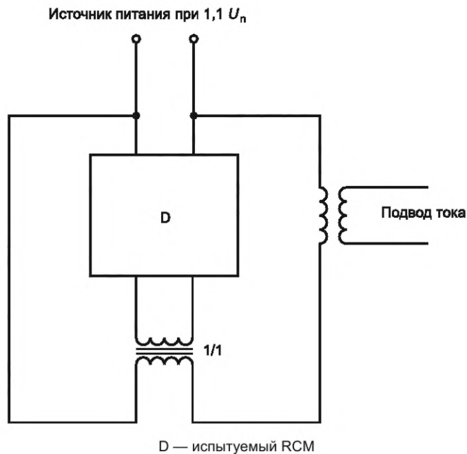
Рисунок 21 — Пример испытательной цепи для проверки старения электронных компонентов (9.21)
