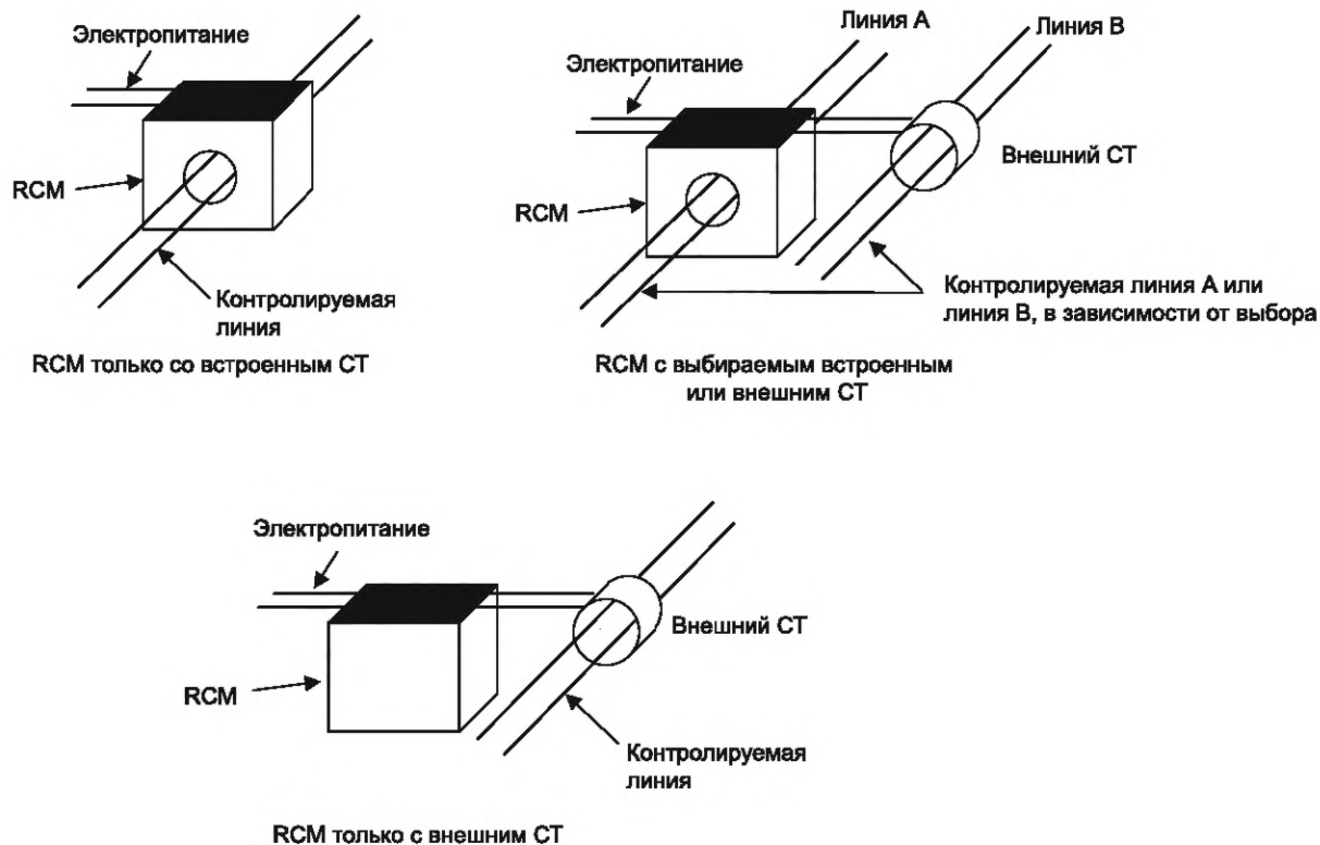
Рисунок 22а — RCMs без подсоединенных контролируемых линий
