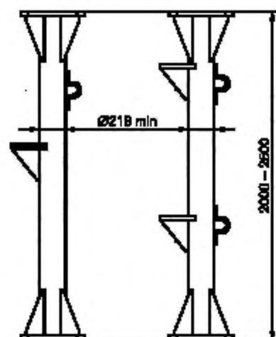
Рисунок 2 — Схема вертикальных опор
