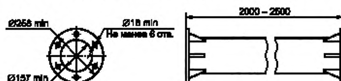
Рисунок 4 — Схема секции горизонтальной опоры
