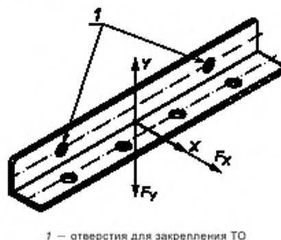
Рисунок 1 — Пример ИдТО и направления сил для проверки прочности
