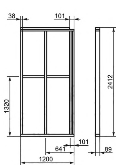
а) Каркас стены А. Сторона 1, зона А
