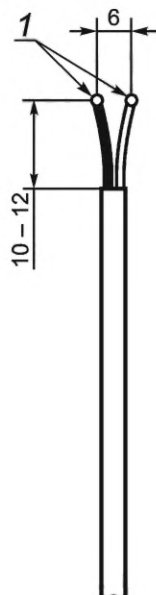
Рисунок С.1 — Метод крепления термоэлемента
