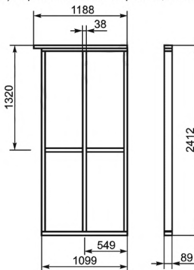
б) Каркас стены В. Сторона 2, зона А
