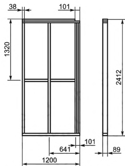
в) Каркас стены С. Сторона 1, зона В
