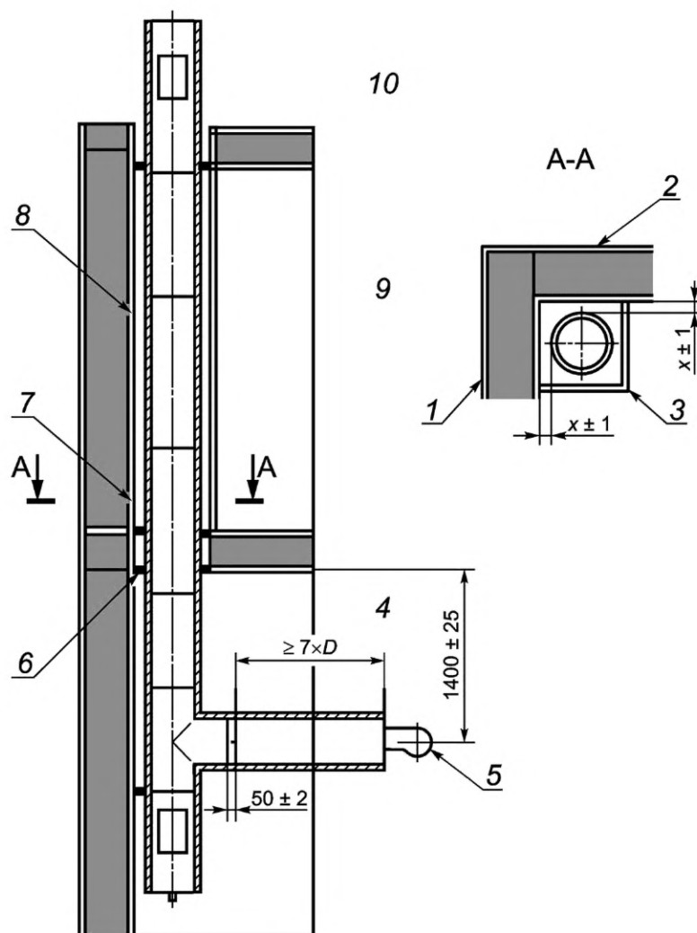
1 — сторона 1; 2 — сторона 2; 3 — оболочка; 4 — зона A; 5 — генератор горячих газов; 6 — противопожарная изоляция; 7 — опора конструкции для удаления дымовых газов; 8 — отверстие; 9 — зона B; 10 — зона C
