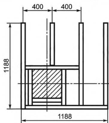
д) Каркас для полов
