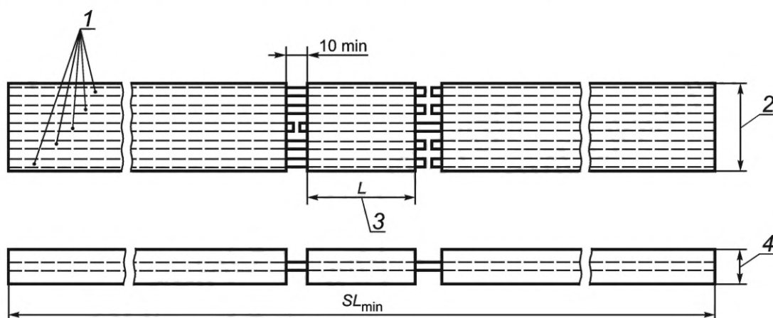
1 — корды основы; 2 — ширина образца; 3 — испытательная длина L ; 4 — толщина образца
