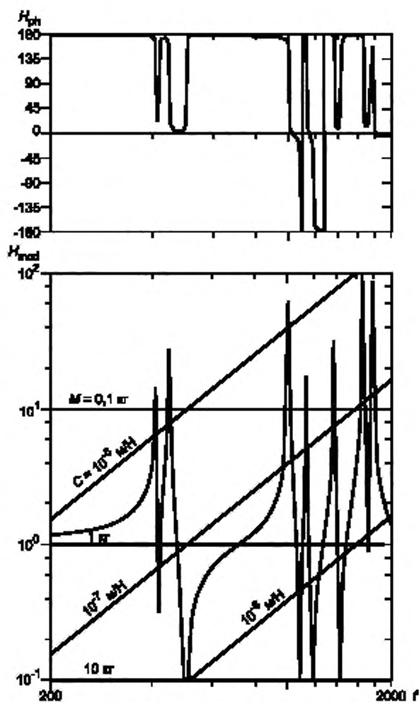
Рисунок 2 — График ускоряемости, соответствующей механической подвижности, изображенной на рисунке 1
