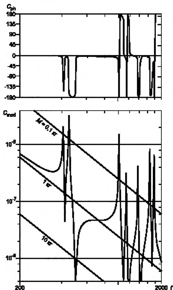
Рисунок 3 — График динамической податливости, соответствующей механической подвижности, изображенной на рисунке 1
