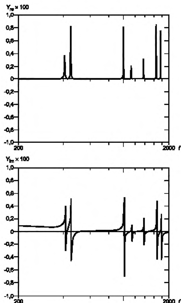
Y_{re} — действительная часть подвижности, m/(H \cdot c) ; Y_{im} — мнимая часть подвижности, m/(H \cdot c) ; f — частота, Гц
