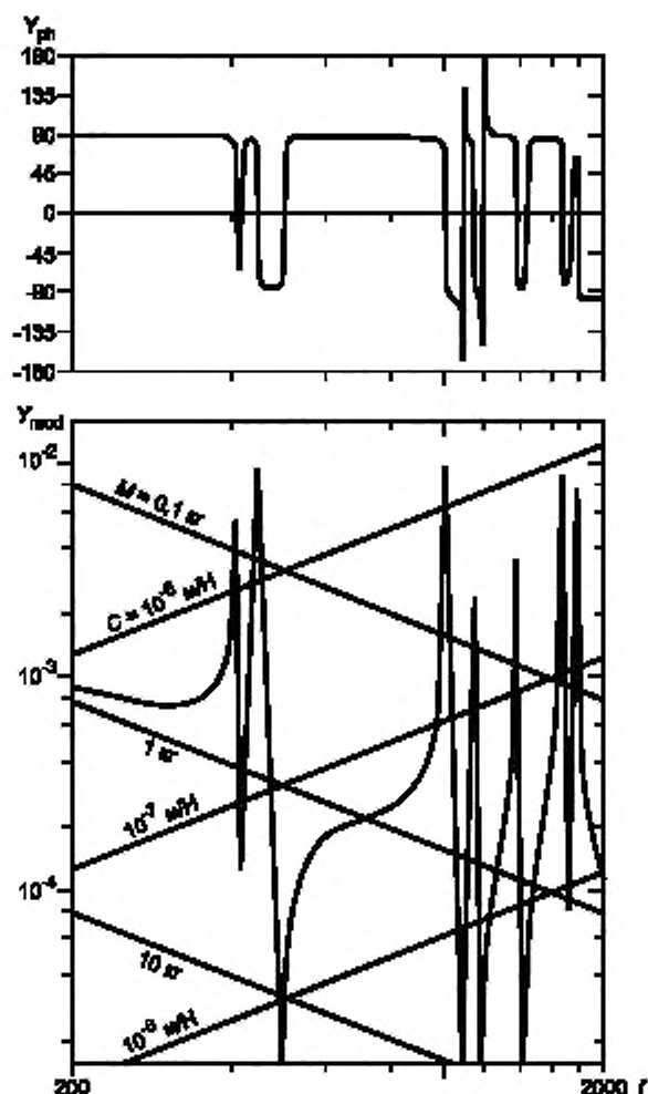
Рисунок 1 — Типичный график механической подвижности, построенный по результатам эксперимента
