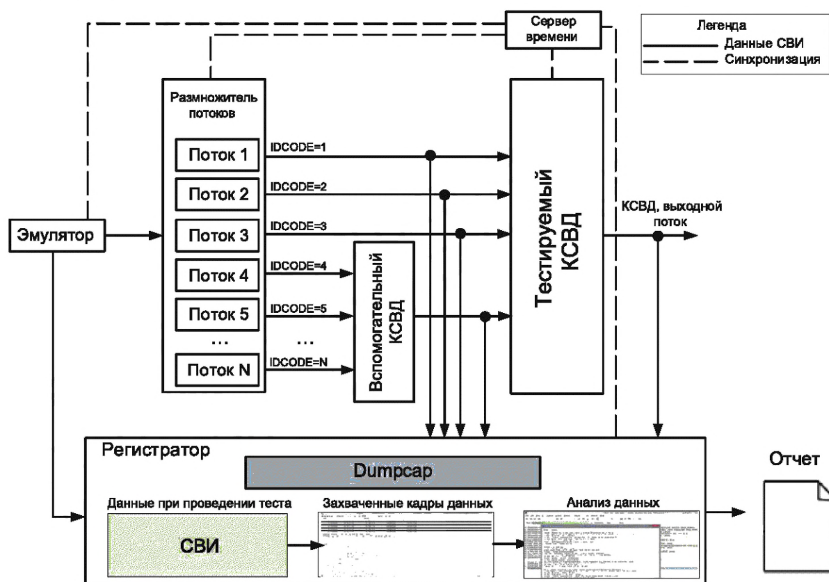
Рисунок В.4 — Схема тестирования режима агрегирования данных
